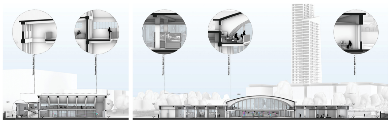
VERTIKALNI PRESECI (1:500) - Poprečni presek 2-2, podužni presek 1-1 (slevo-nadesno)
