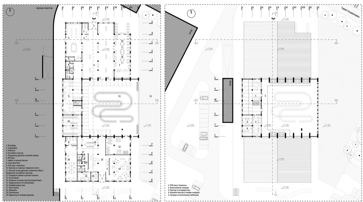
OSNOVE ETAŽA (1:500) - Osnova prizemlja, osnova galerije (slevo-nadesno)
