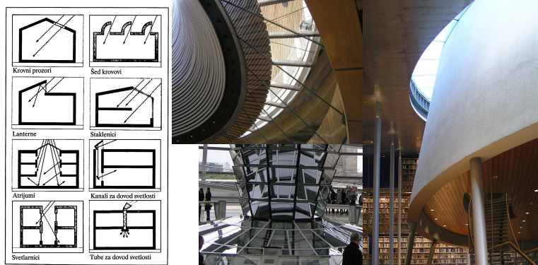
Slika 5. Tipovi (levo, Krstić-Furundžić, 2006) i primeri (desno) struktura za uvođenje dnevne svetlosti u zone zgrade udaljene od fasada. Primeri: The Senedd, Cardiff , gore; TU Delft biblioteka, sredina; Reichstag , Berlin, dole. Izvor: Autor
