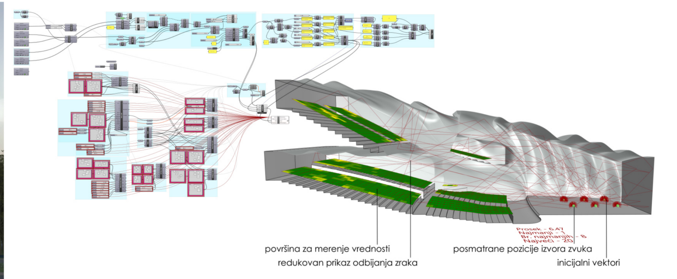
ALGORITAM ZA GENERISANJE FORME KONCERTNE DVORANE I PROVERU AKUSTIČNIH PERFORMANSI ▼
