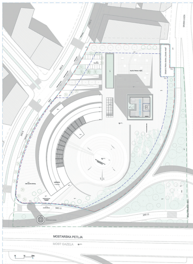
СИТУАЦИОНИ ПЛАН СА ОСНОВАМА КРОВА, Р 1:500
