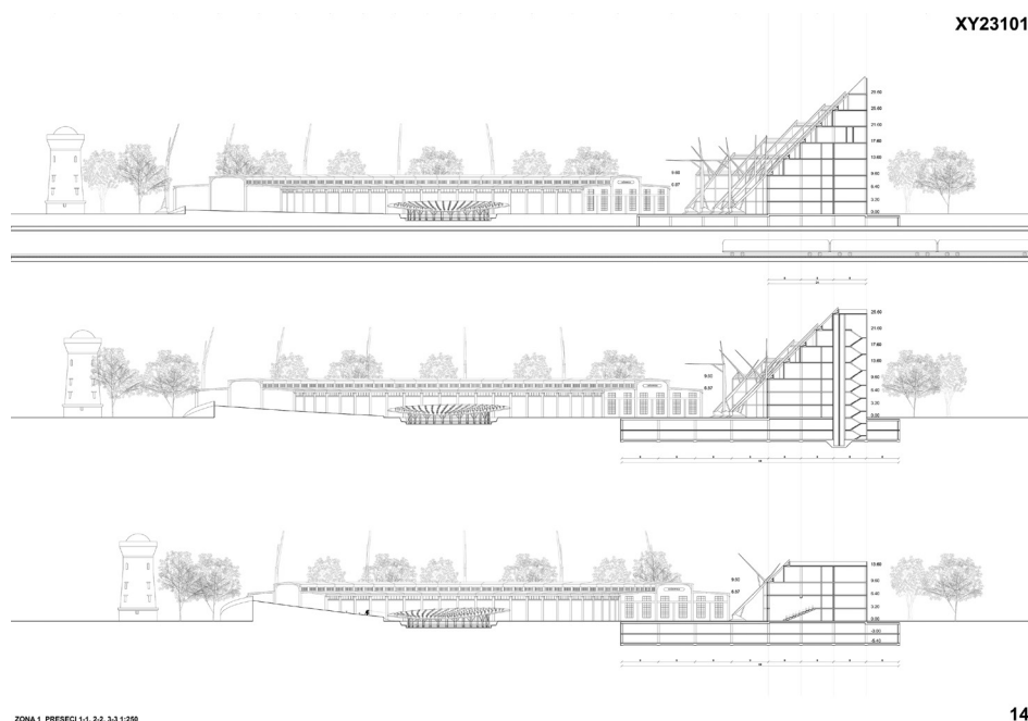
ZONA 1_PRESECI 1-1, 2-2, 3-3 1:250
