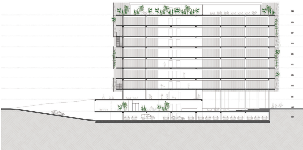
ЗОНА 1. ОБЈЕКАТ АНЕКСА - ПОДУЖНИ ПРЕСЕК 1-1, 1:250
