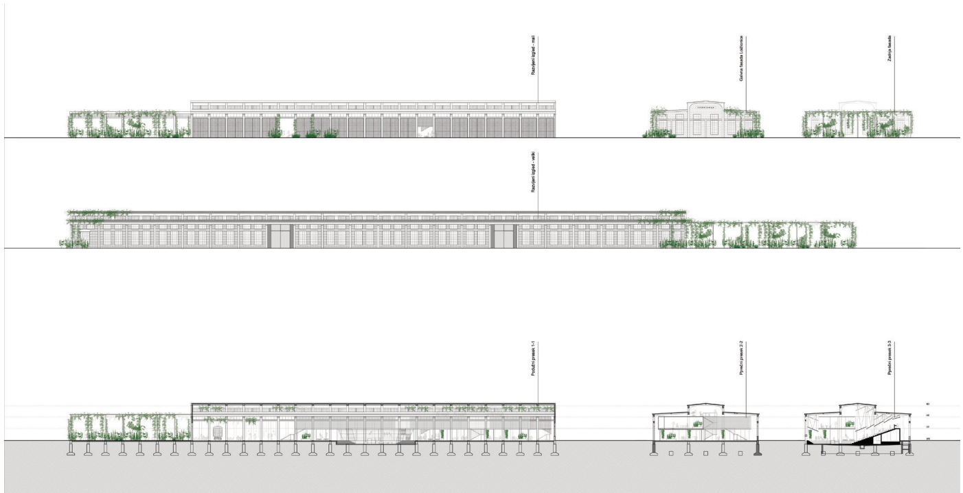
ЗОНА 1. ОБЈЕКАТ ЛОЖИОНИЦЕ - КАРАКТЕРИСТИЧНИ ПРЕСЕЦИ И РАЗВИЕНИ ИЗГЛЕДИ, 1:250
