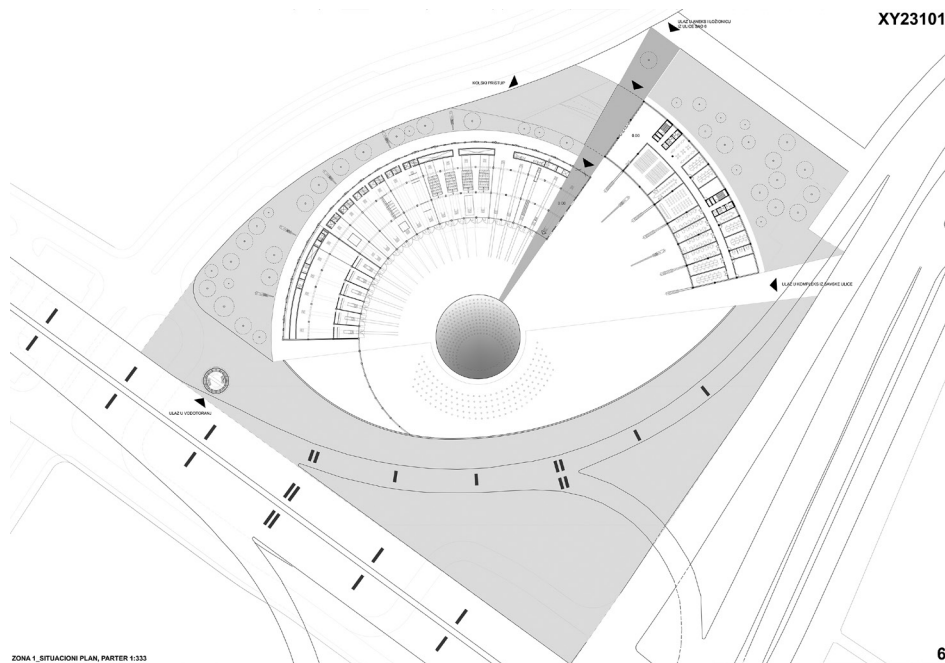
ZONA 1_SITUACION PLAN, PARTER 1:333
