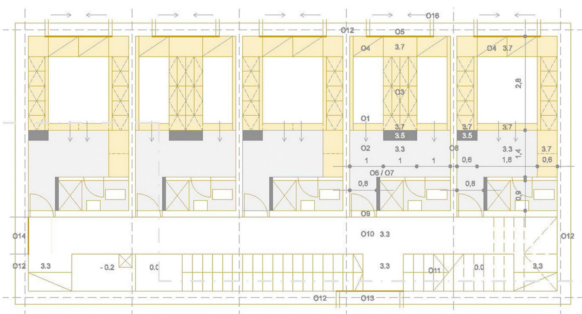
Osnova sprata
