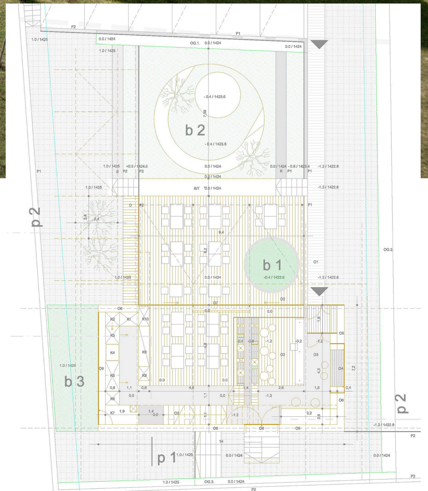
Osnova prizemlja
