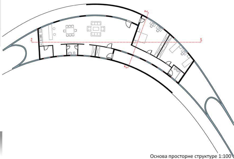
Основа просторне структуре 1:100
