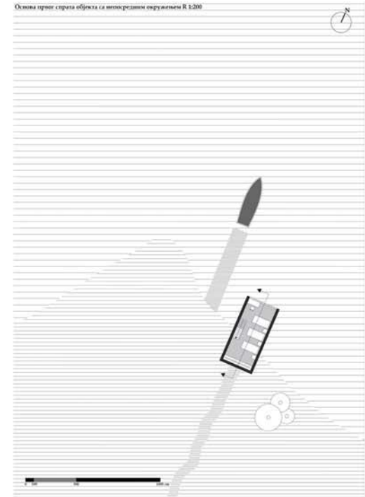
Основа првог спрата објекта са непосредним окружењем R 1:200
