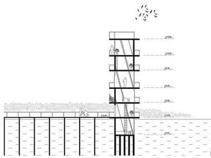
изглед
