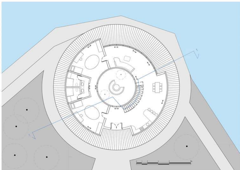
основа приземља објекта
