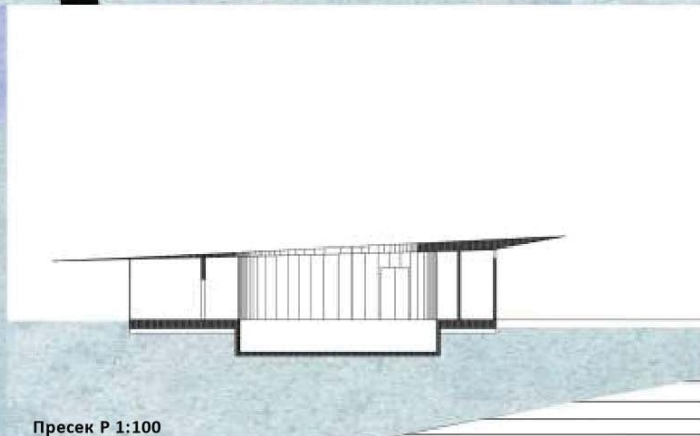
Пресек P 1:100
