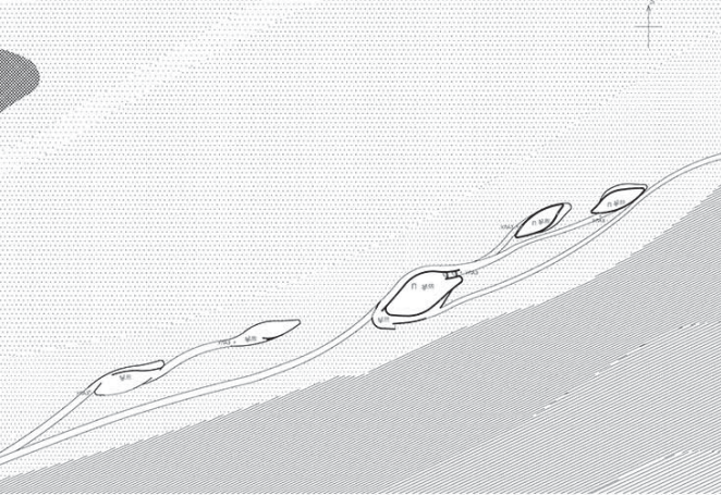
Ситуација Р 1:500
