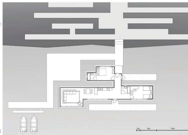
Основа, функционално решење
