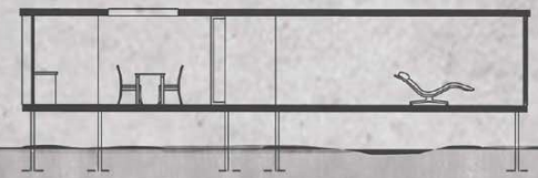
ПРЕСЈЕК СТРУКТУРЕ Р 1:100
