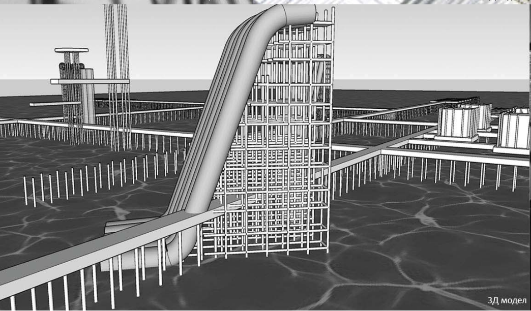
Кадар макете
