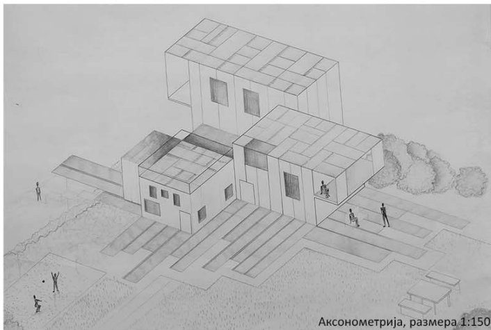
Аксонometriја, размера 1:150
