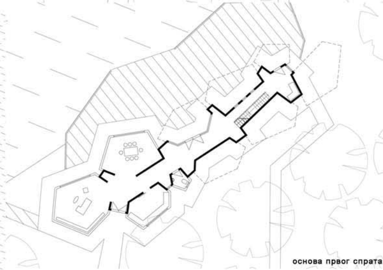
основа другог спрата
