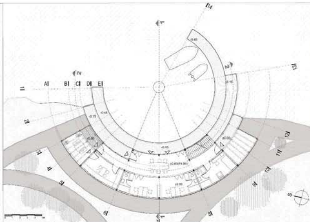
Osнова prizemlja
