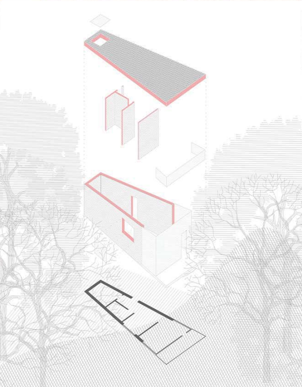
ЕКСПЛОДИРАНА АКСОНОМЕТРИЈА
