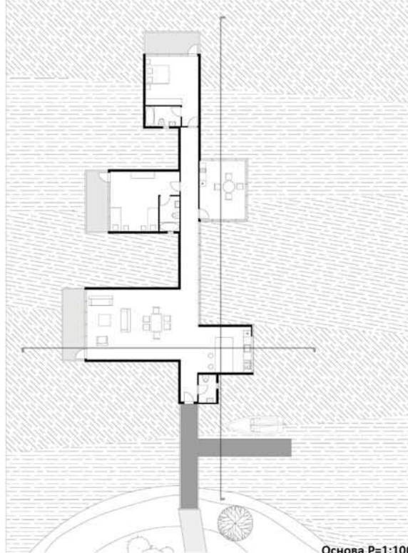
Основа Р=1:100
