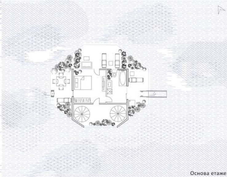
Основа етаже
