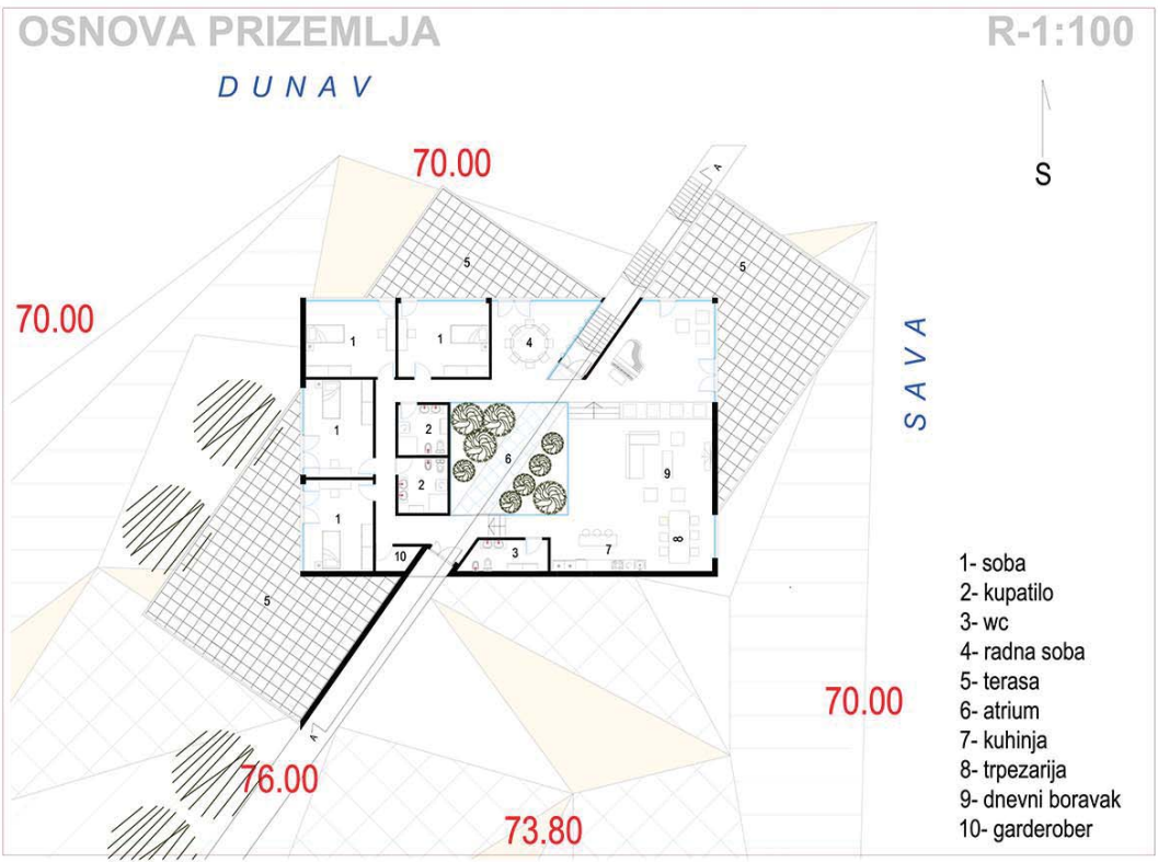
OSNOVA PRIZEMLJA R-1:100
