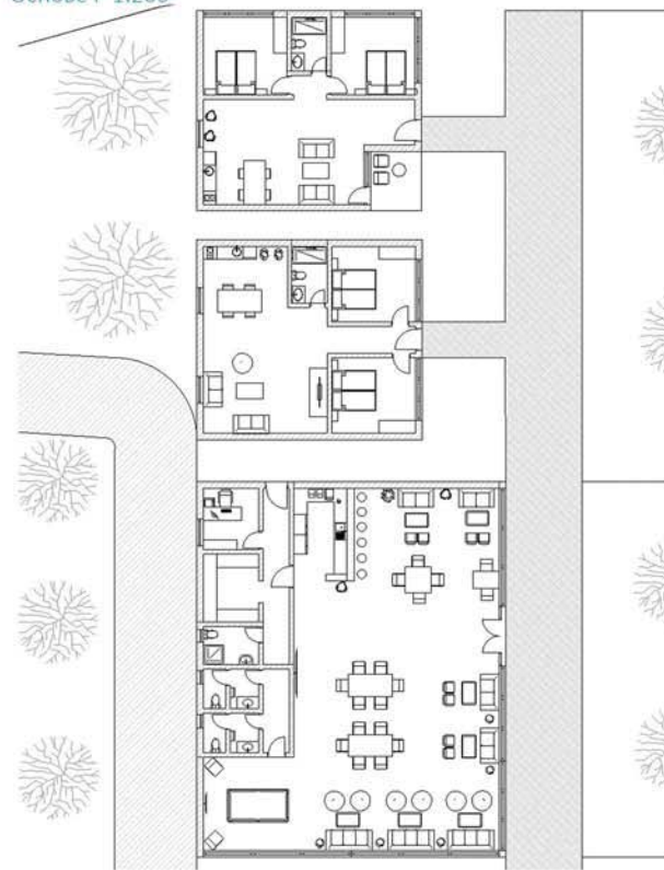
Основе Р 1:200
