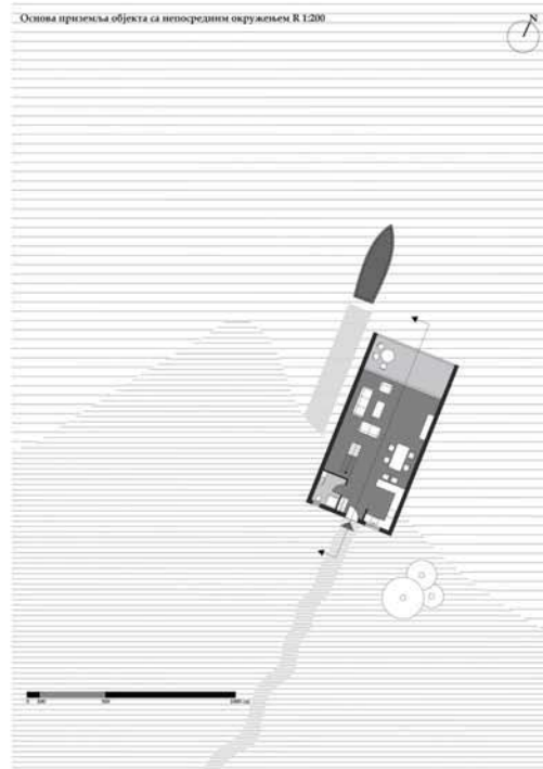
Основа приземља објекта са непосредним окружењем R 1:200
