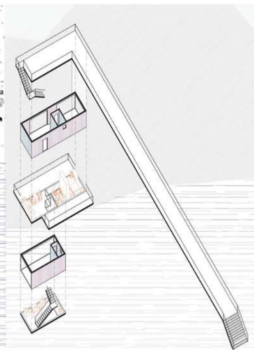
развијена аксонометрија
