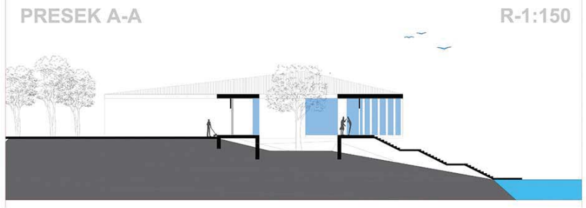
PRESEK A-A R-1:150
