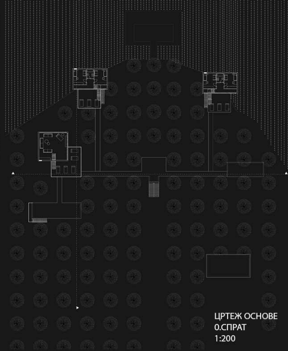
ЦРТЕЖ ОСНОВЕ 0. СПРАТ 1:200
