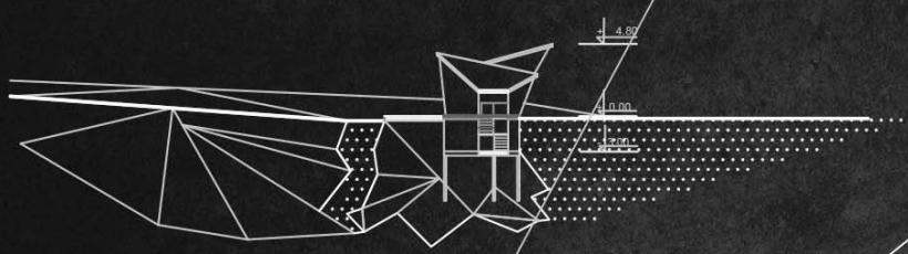
ПРЕСЕК 1-1 Р 1:200
