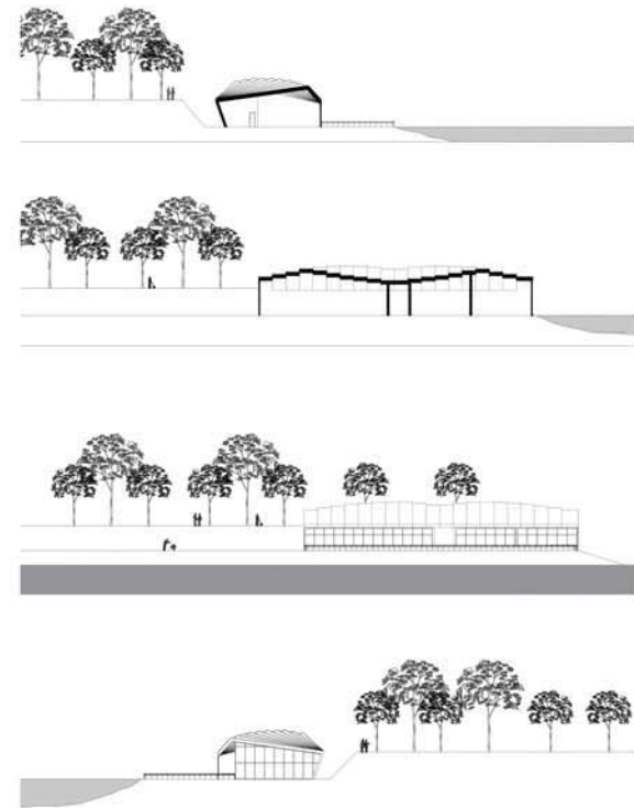
Пресеци и изгледи Р 1:200
