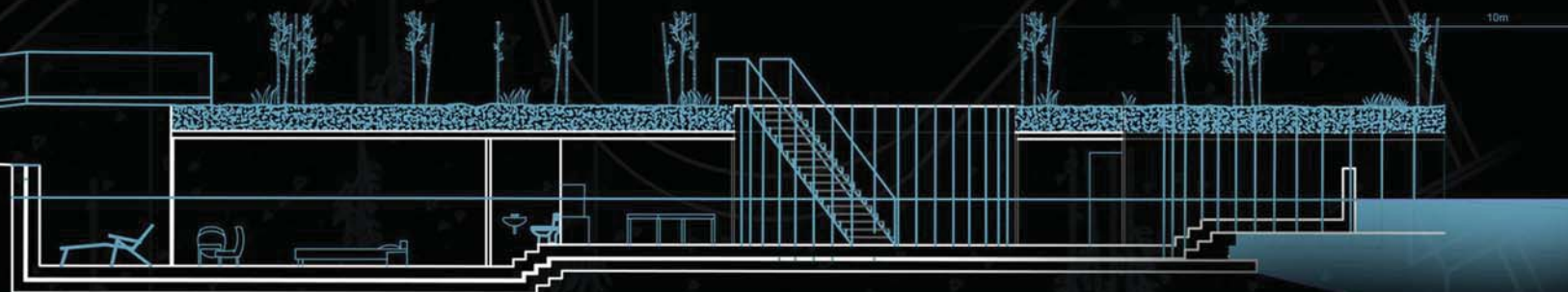
ПРЕСЕК ОБЈЕКТА
