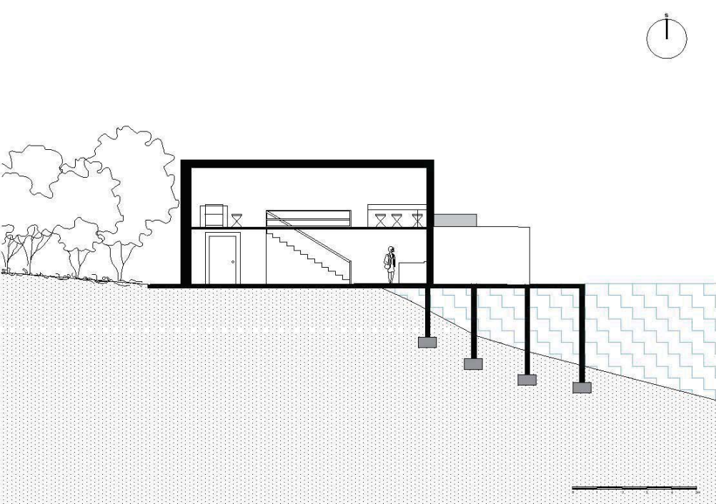
Пресек куће на ушћу
