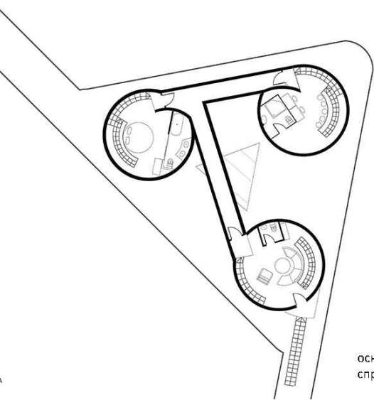
изглед 1:100
