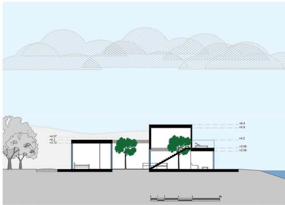
пресек 1 - 1 објекта
