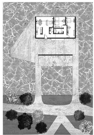
Основа 1:100
