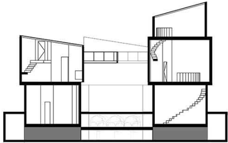
попечни пресек 1:100
