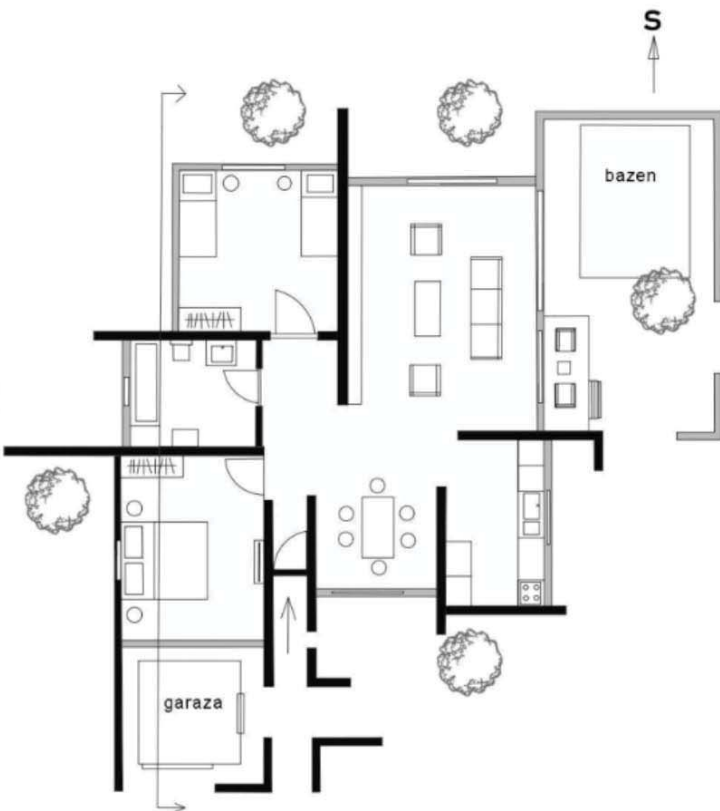
основа 1:200
