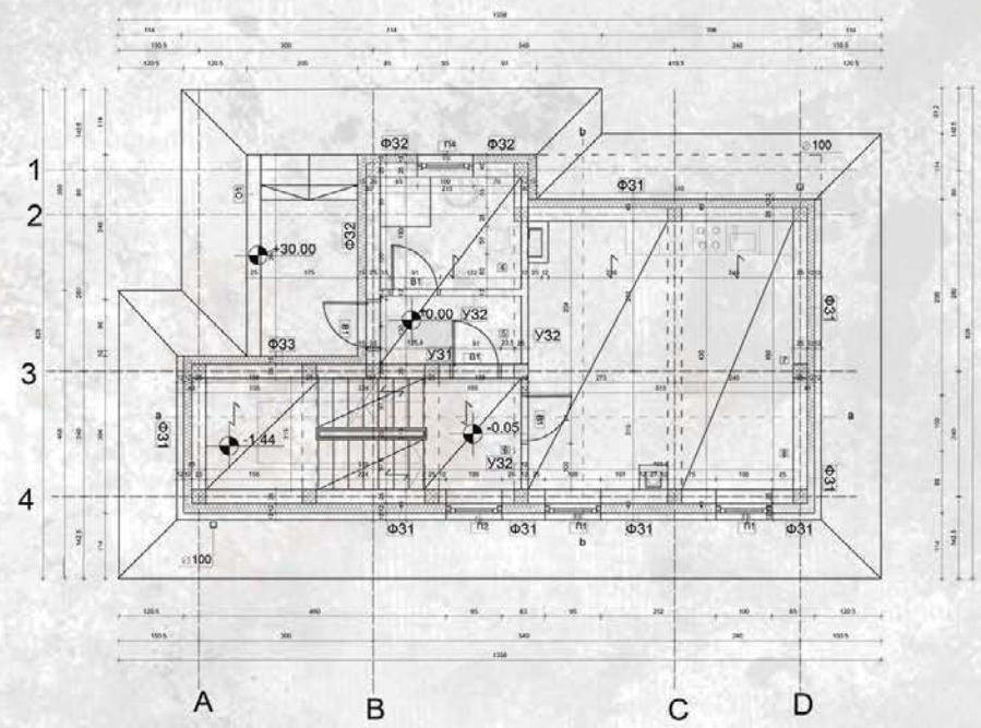
Основа приземља
