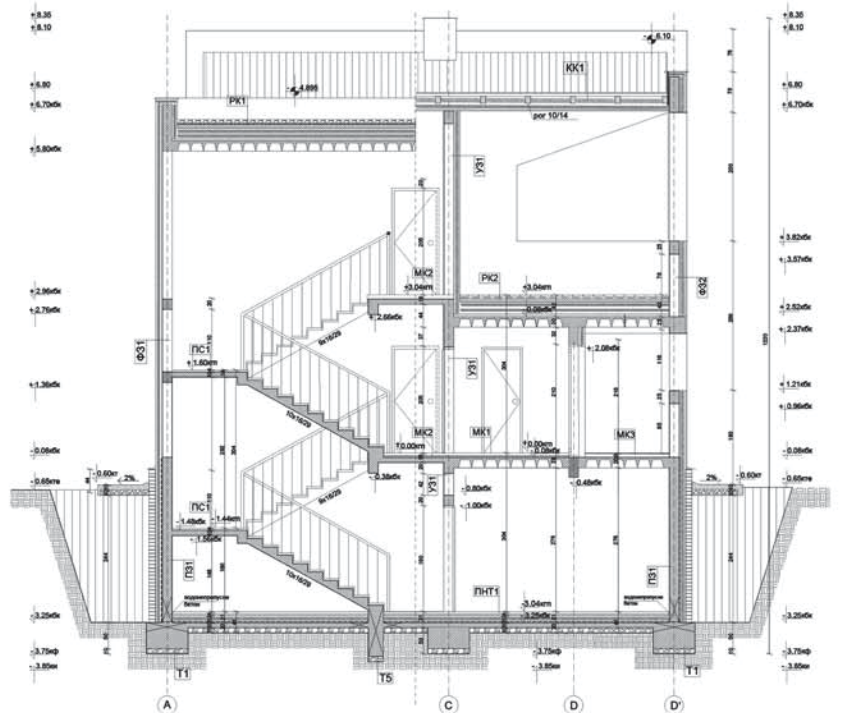
ПОДУЖНИ ПРЕСЕК А-А
