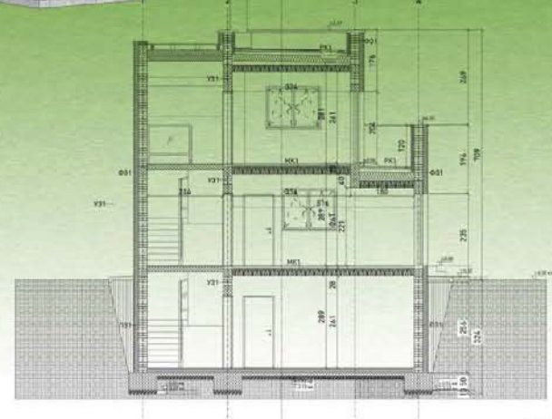
пресек Б-Б
