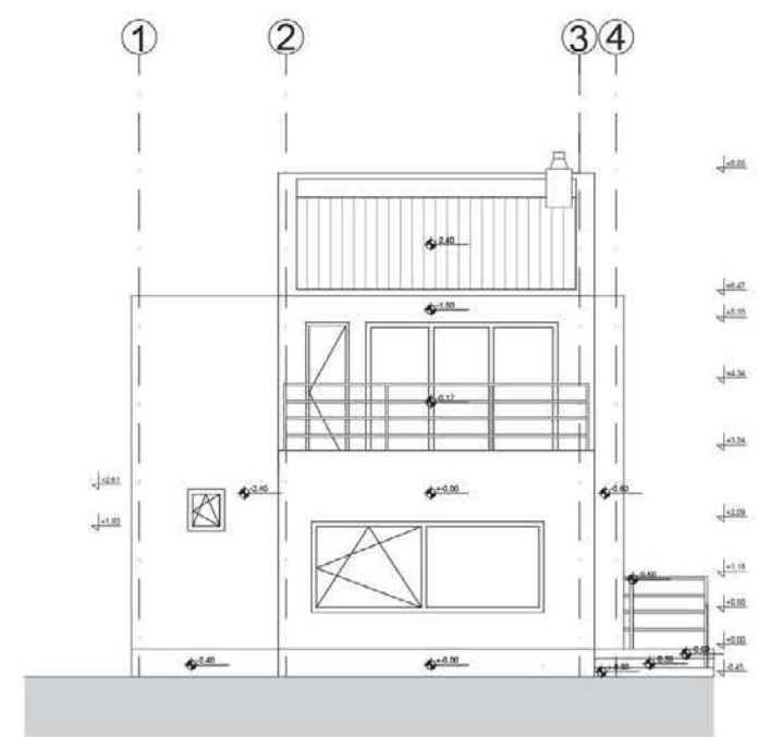
Пресек а - а Изглед 2
