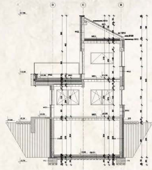
Пресек С-С
