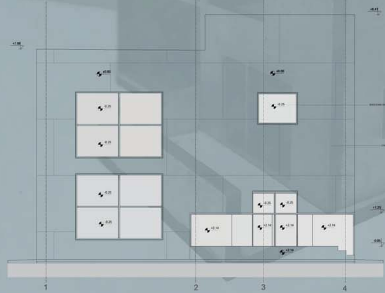
изглед 2
