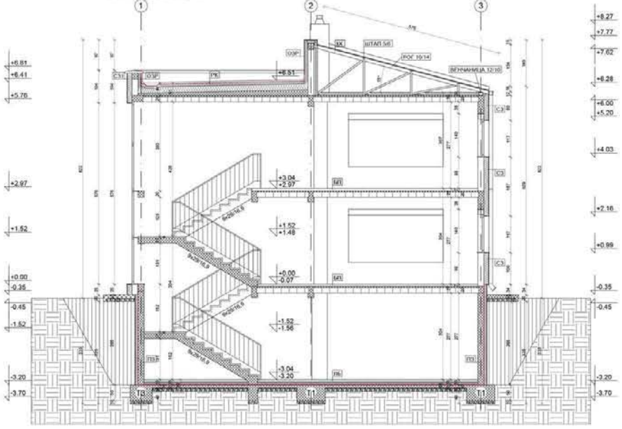
ПРЕСЕК Б-Б
