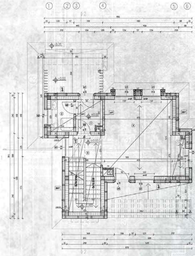
основа приземља
