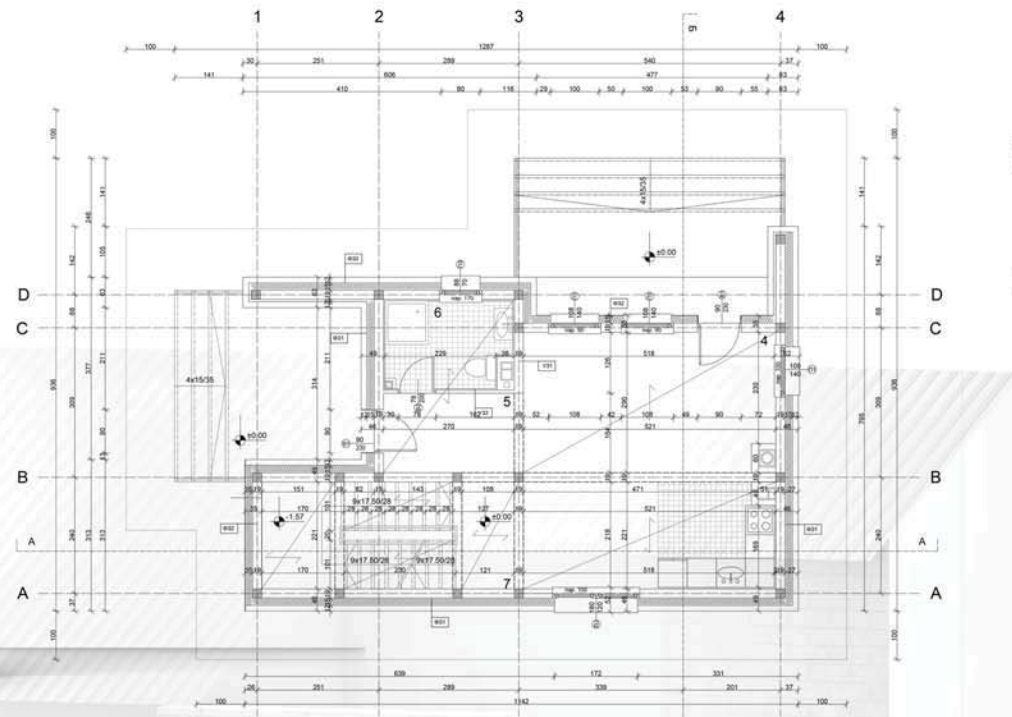
Основа приземља
