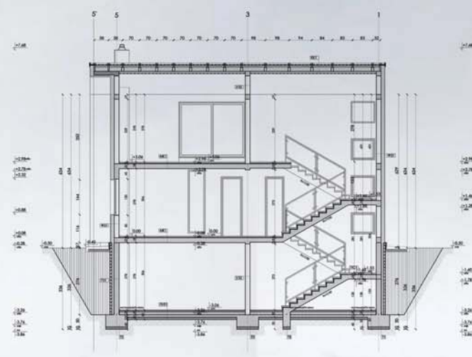
пресек 1-1
