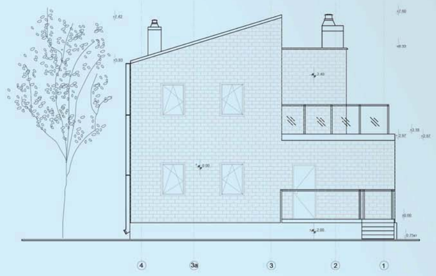
ИЗГЛЕД
