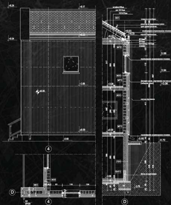
Детаљ
