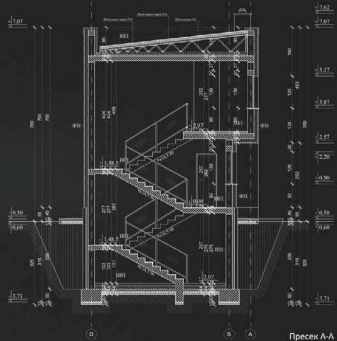
Пресек А-А
