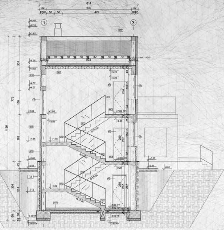
Пресек 2 - 2
