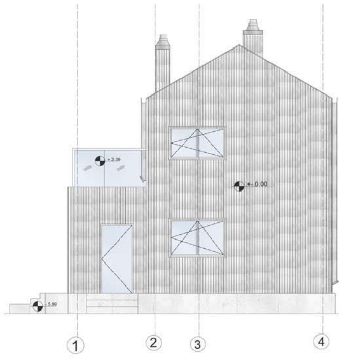
МАТЕРИЈАЛИЗОВАНИ ИЗГЛЕД
