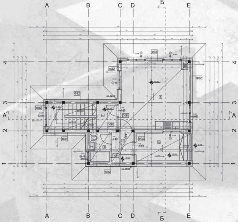
основа приземља
