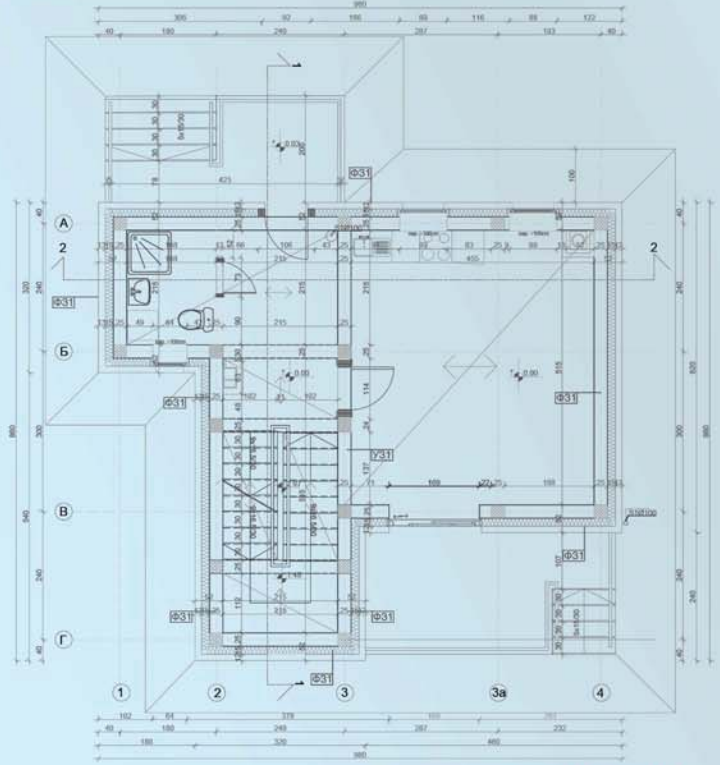
ОСНОВА ПРИЗЕМЉА
