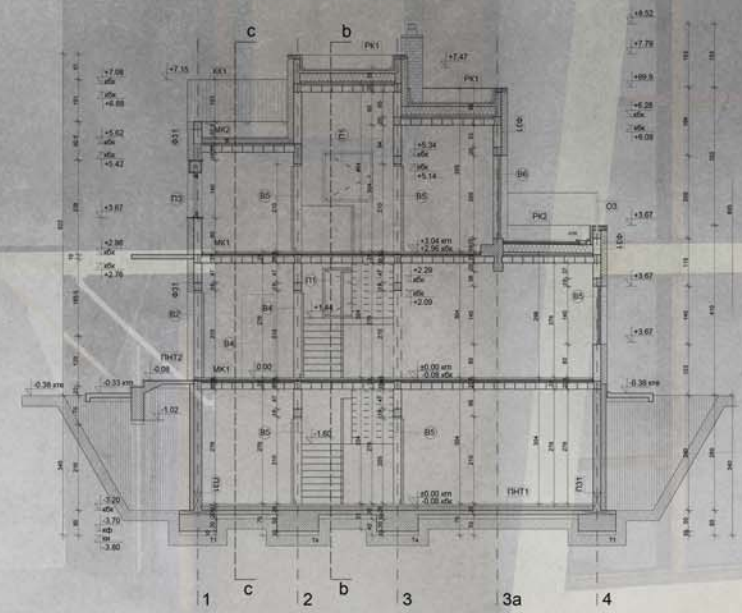
ПРЕСЕК А-А
