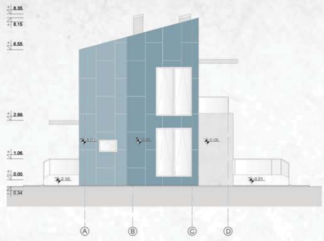
изглед 3
