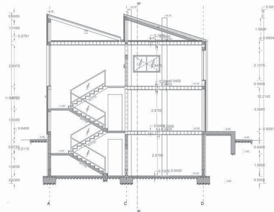
подужни пресек а_а
