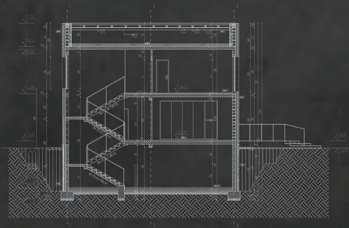
ПРЕСЕК А-А
