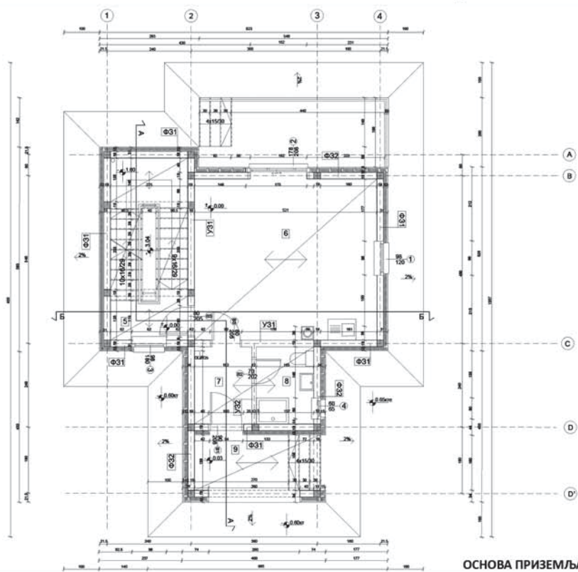
ОСНОВА ПРИЗЕМЉА
