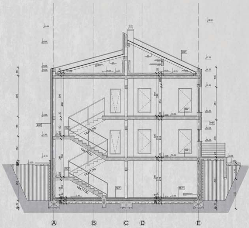
Подужни пресек а-а
