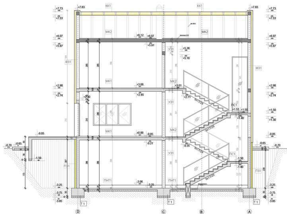
Пресек А-А
