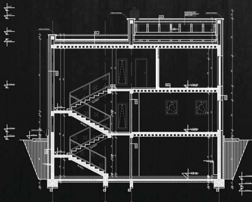
ПОДУЖНИ ПРЕСЕК b-b
