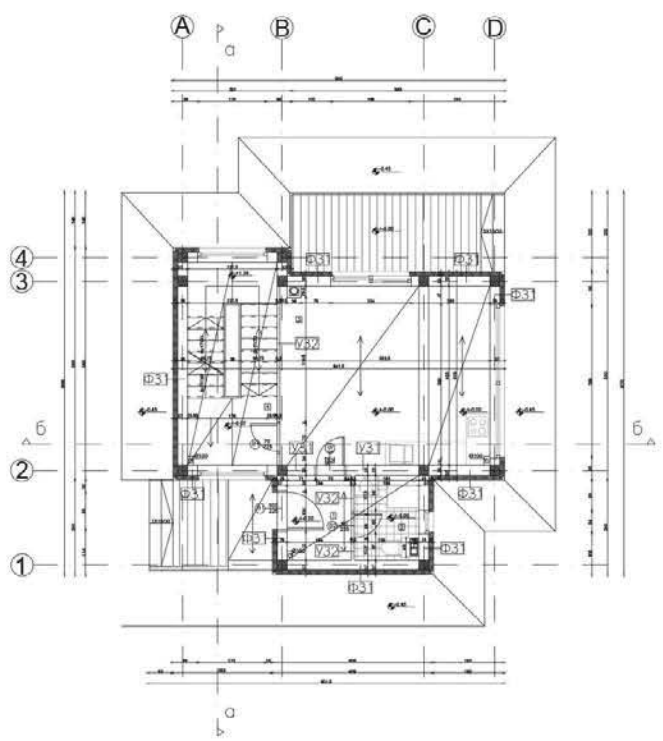
Основа приземља Изглед 1
