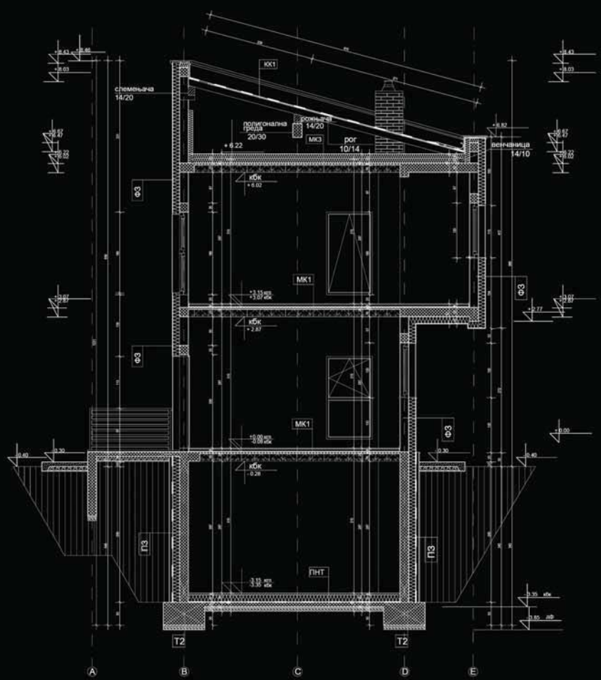
ПОПРЕЧНИ ПРЕСЕК 2-2
