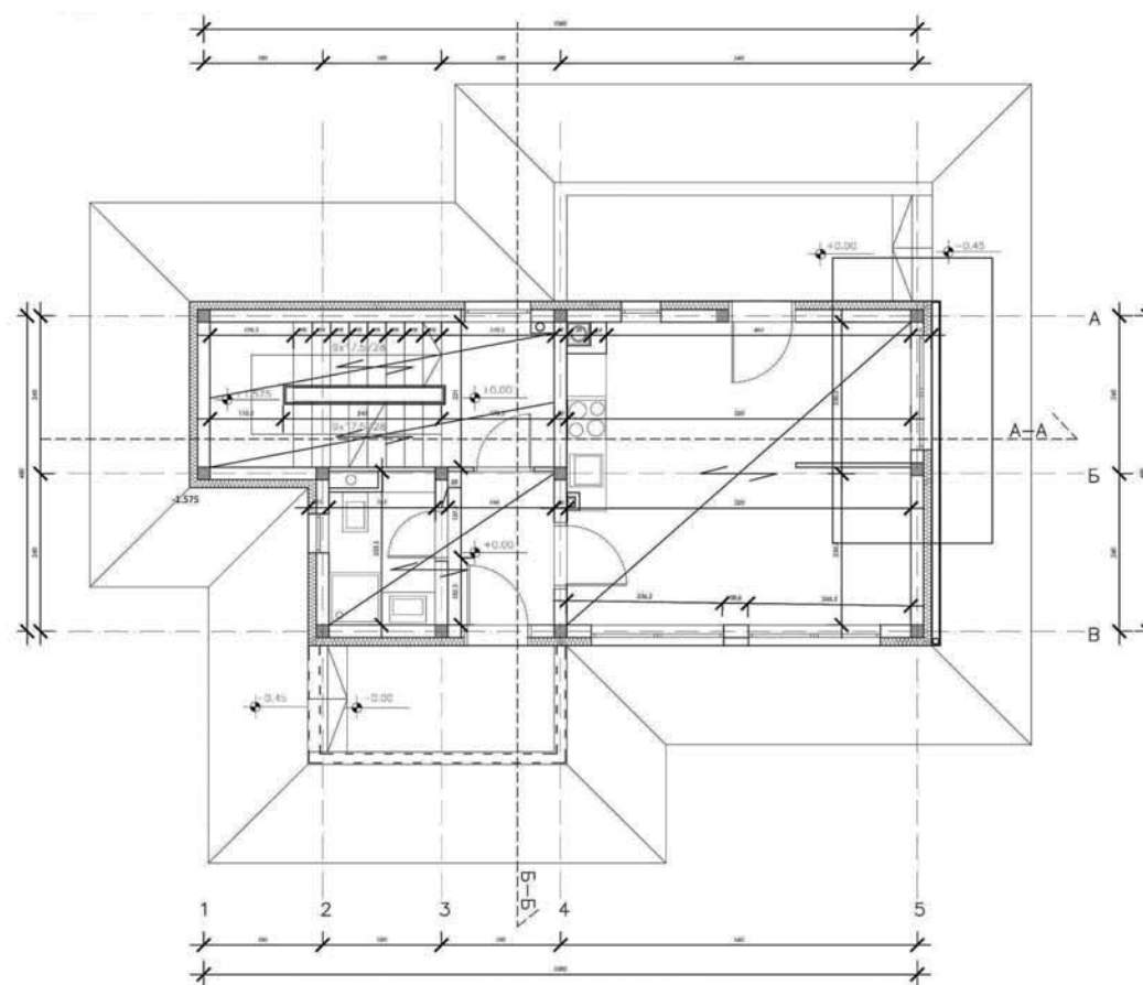
ОСНОВА ПРИЗЕМЉА
