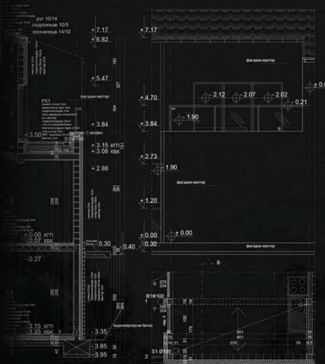
ДЕТАЉ ФАСАДЕ
