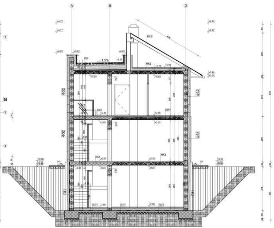
Пресек а-а
