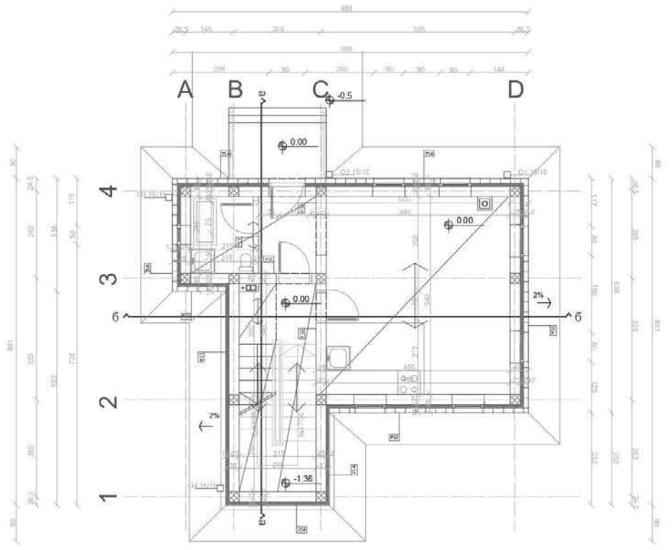
Основа приземља
