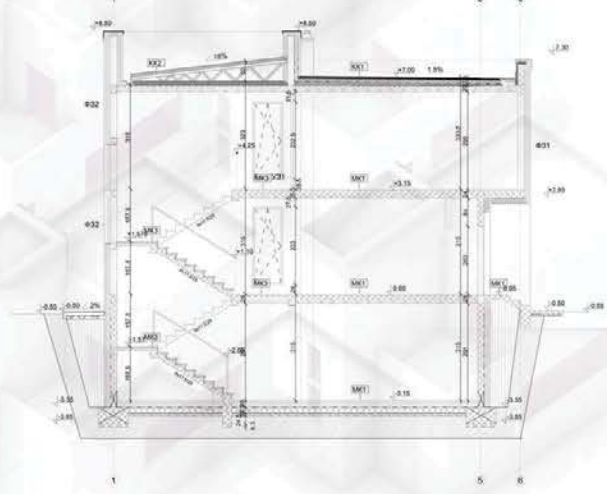
ПОПРЕЧНИ ПРЕСЕК А-А
