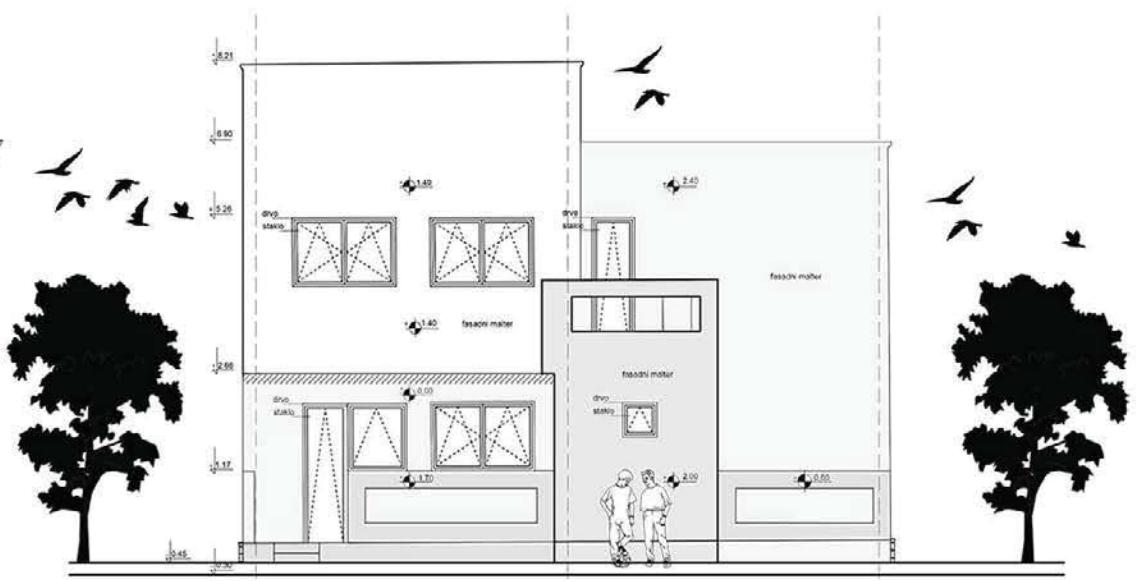
Изглед са предње стране
