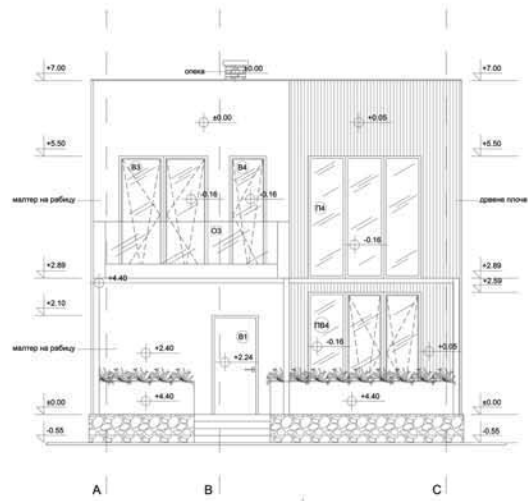
ИЗГЛЕД 3
