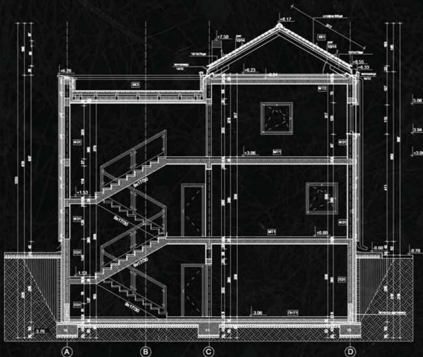
Пресек Б-Б
