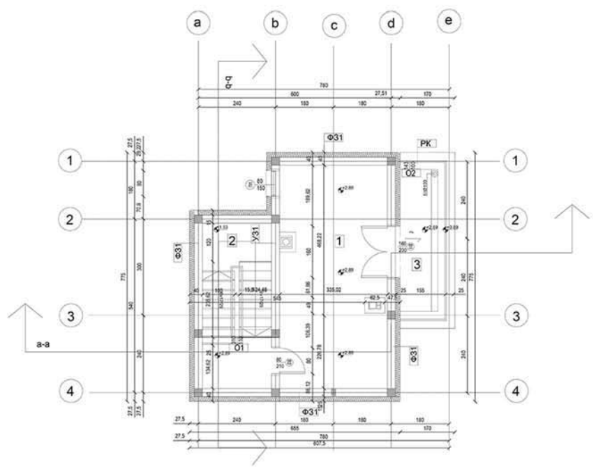
ОСНОВА ПРИЗЕМЉА
