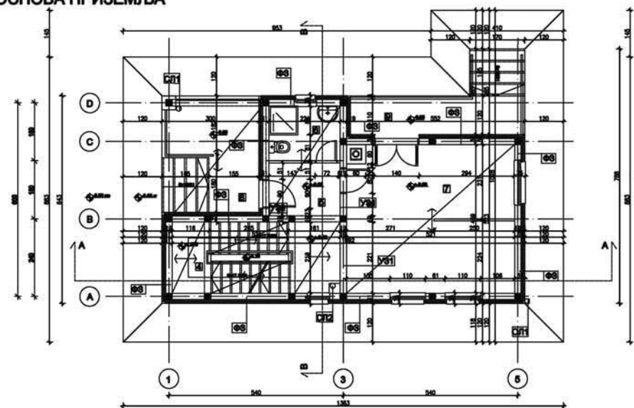
ОСНОВА ПРИЗЕМЉА
