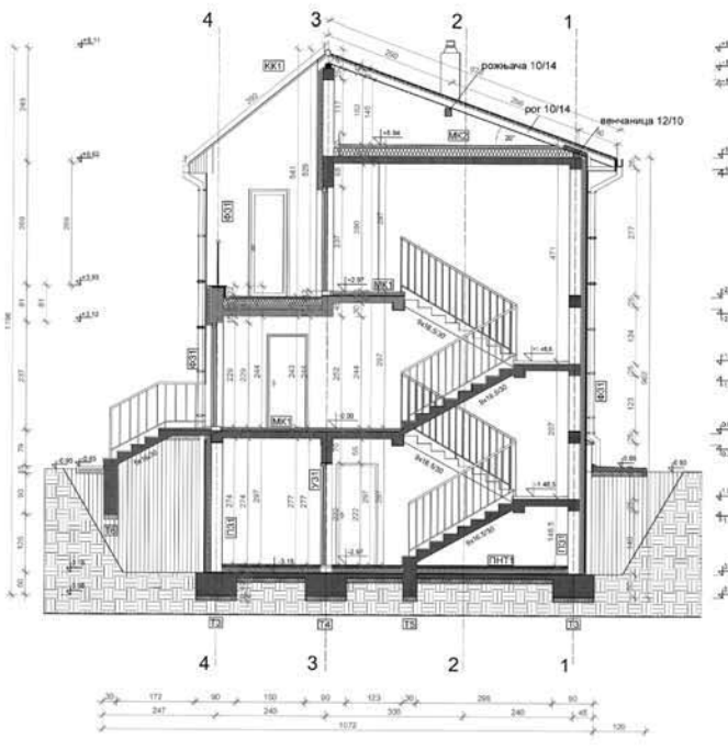
Пресек а-а
