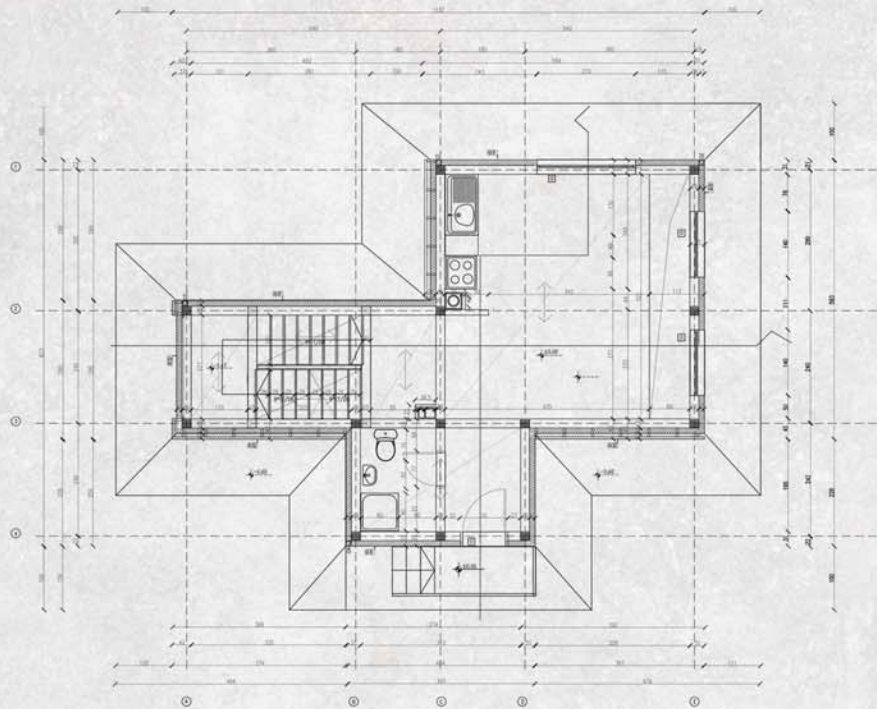
Основа приземља
