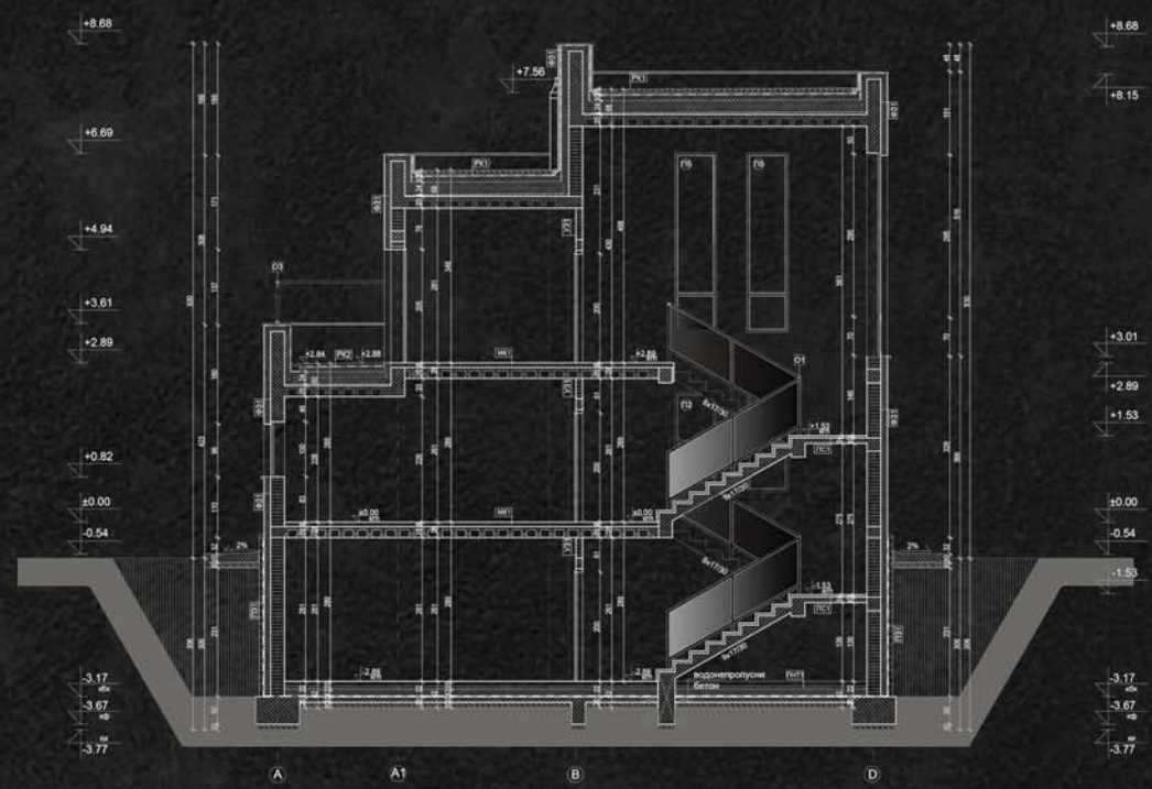
подужни пресек А-А
