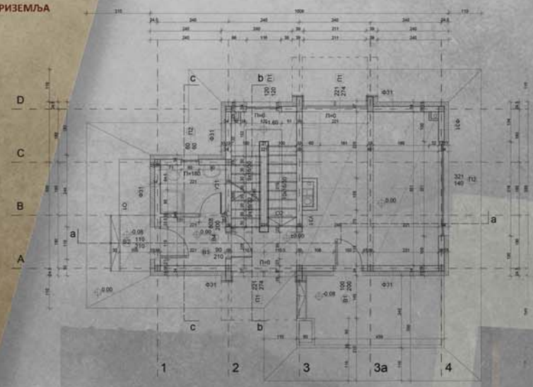
ОСНОВА ПРИЗЕМЉА
