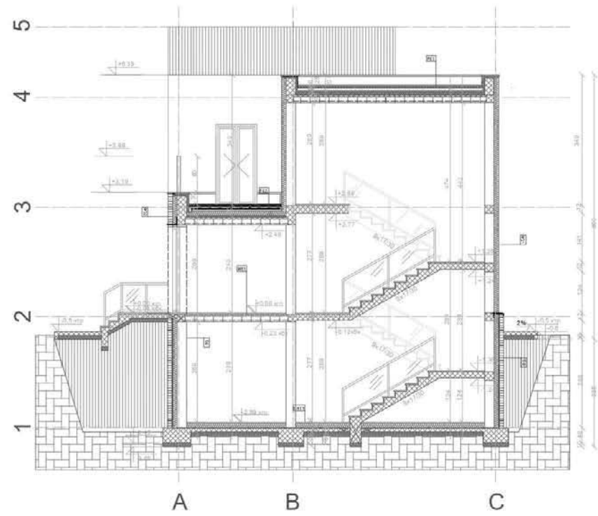
Пресек а-а
