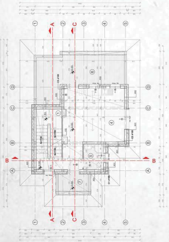
основа приземља
