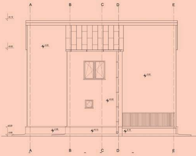
IZGLLED 1
