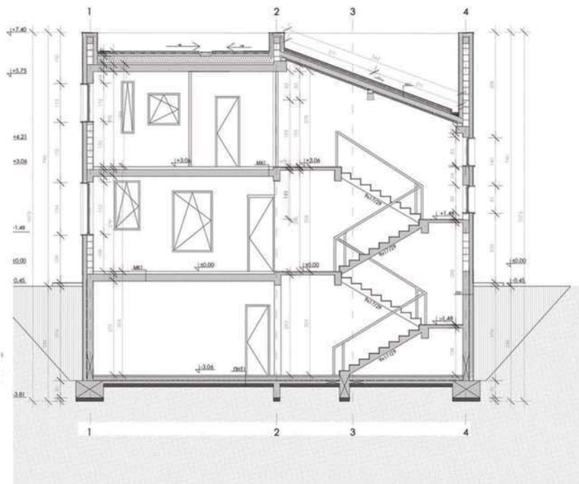
ПРЕСЕК "а-а"
