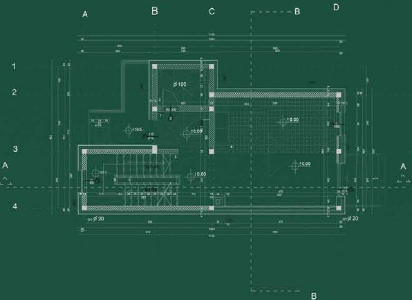
ОСНОВА ПРИЗЕМЉА
