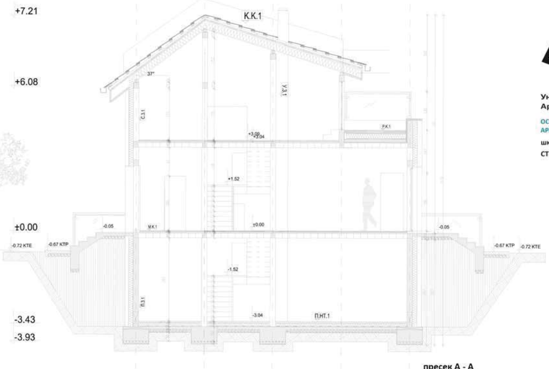
пресек А - А
