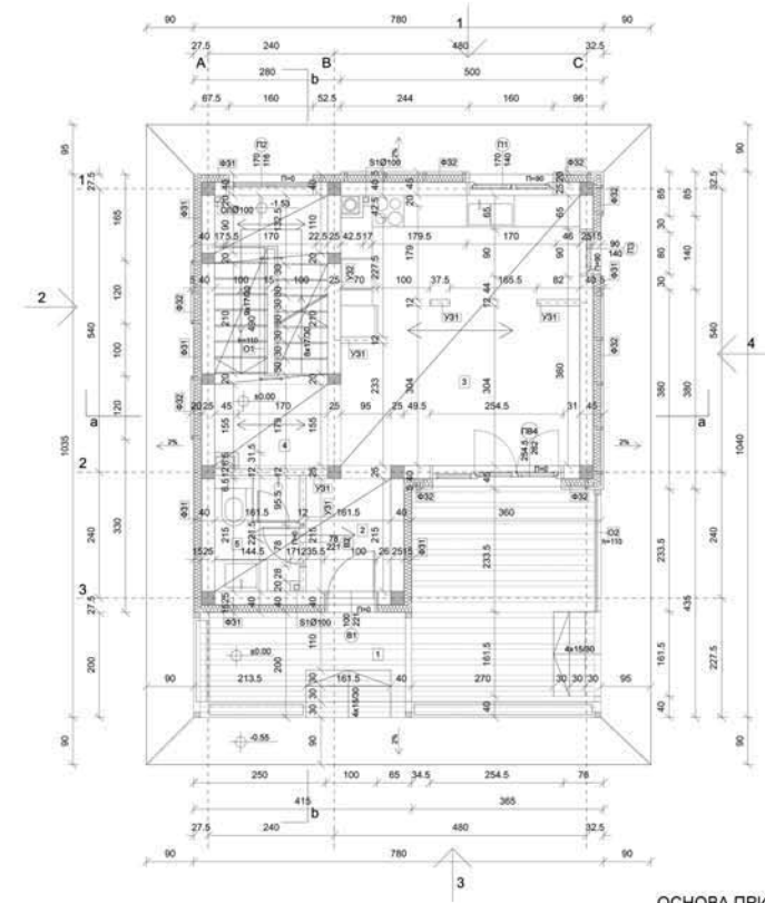
ОСНОВА ПРИЗЕМЉА
