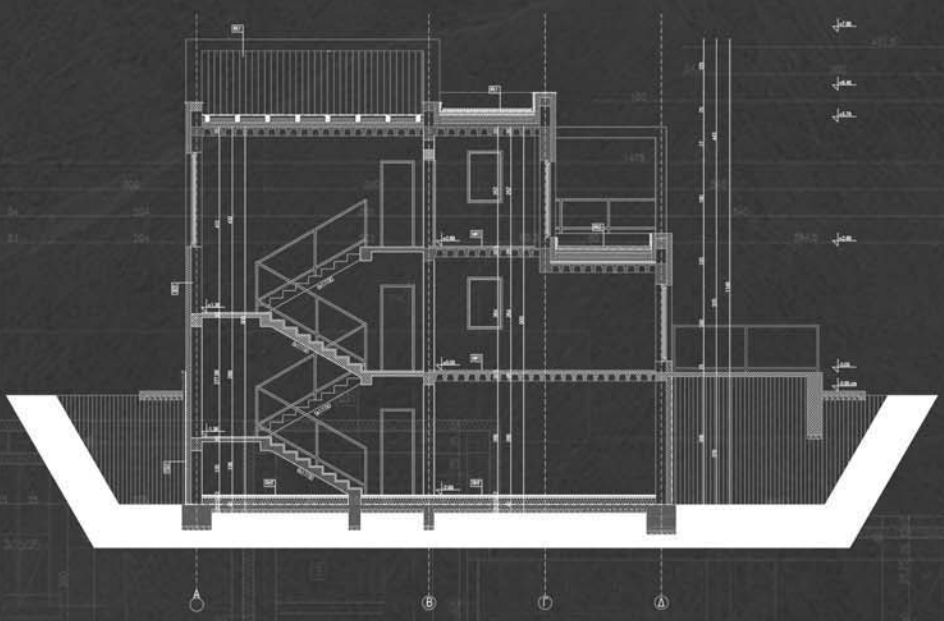
Пресек 1-1
