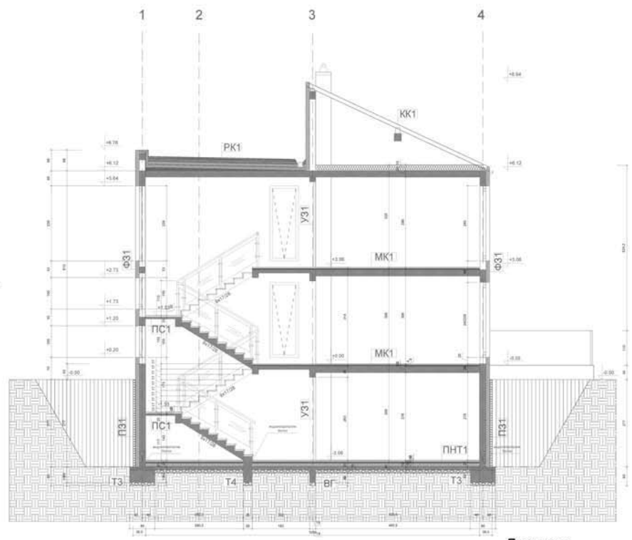
Пресек а-а
