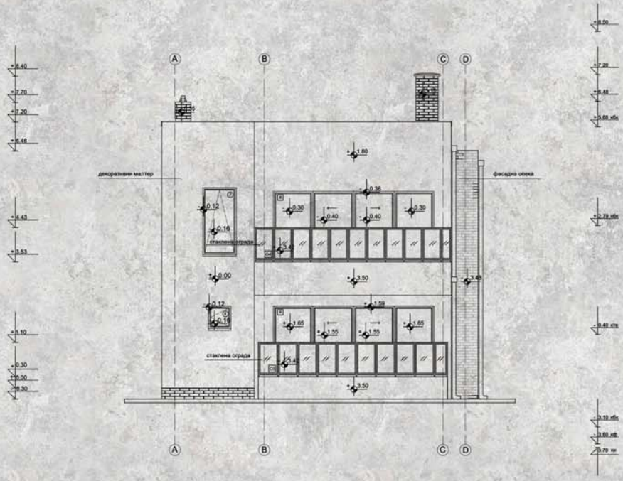
изглед
