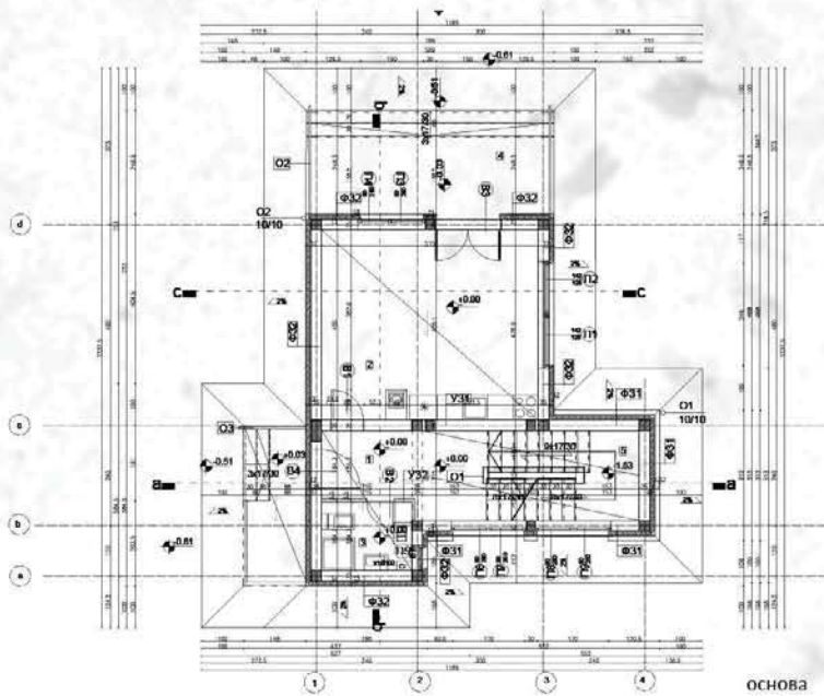
ОСНОВА
