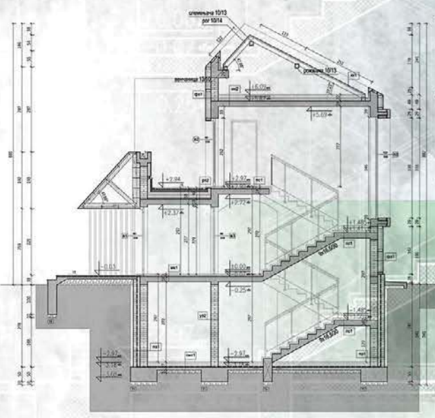
пресек 2-2
