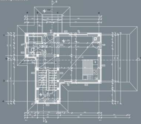
Основа приземља
