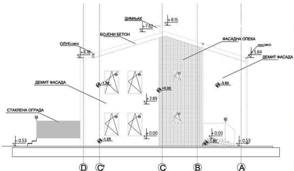
Изглед 1
