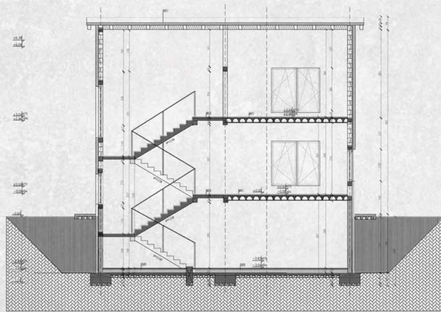
Подужни пресек
