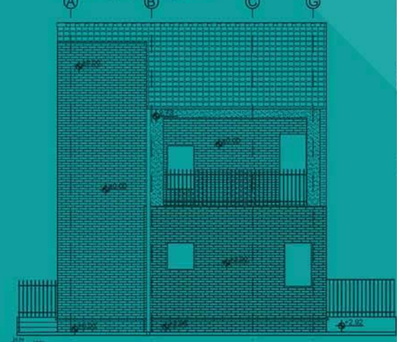
Изглед фасаде 3
