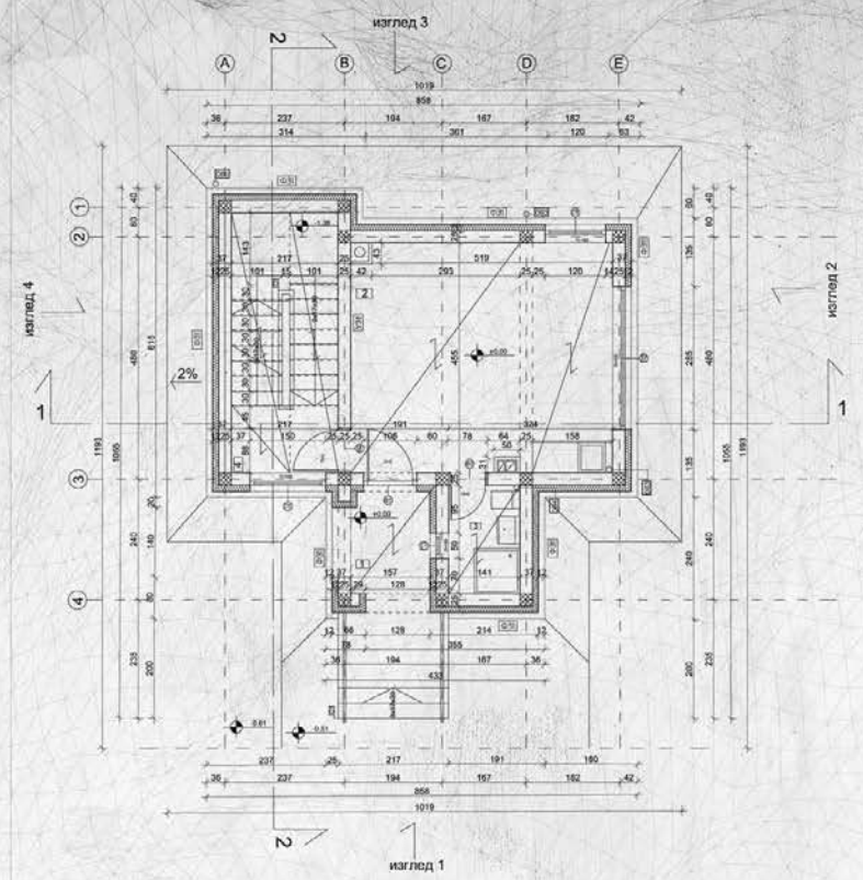
Основа приземља
