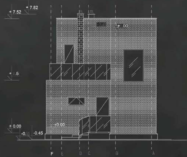
БОЧНА ФАСАДА
