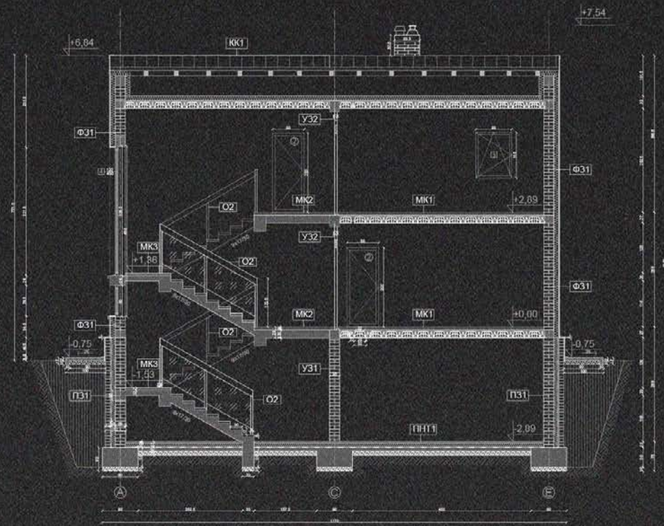
ПРЕСЕК 2-2
