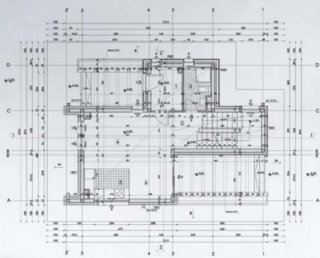
основа приземља
