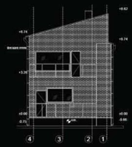
ИЗГЛЕДИ
