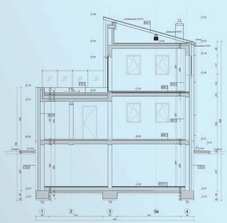
ПРЕСЕК 2-2
