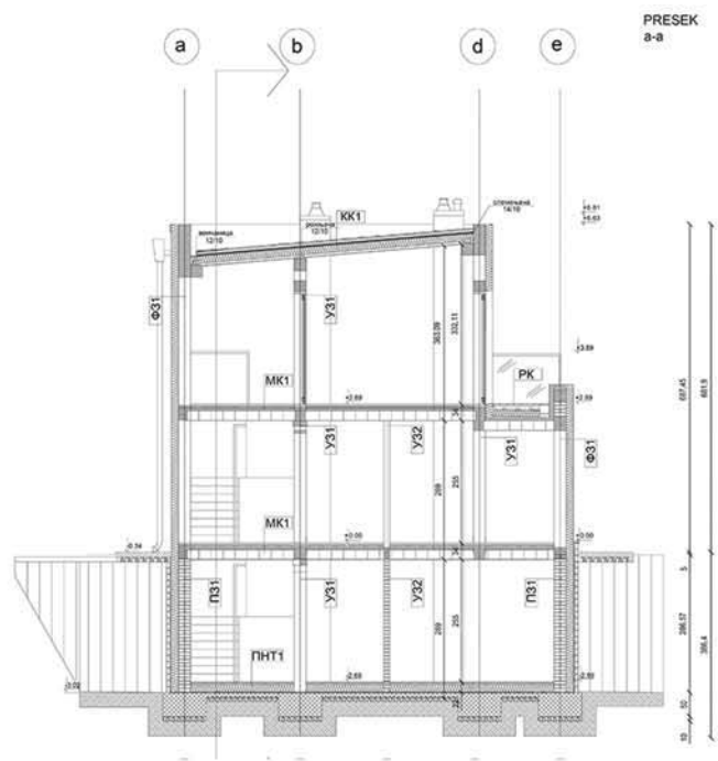
ПРЕСЕК
