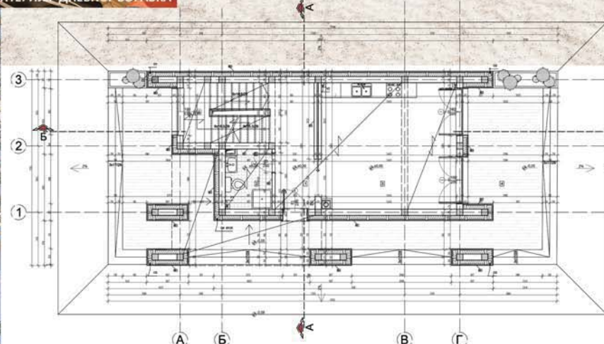
ОСНОВА ПРИЗЕМЉА
