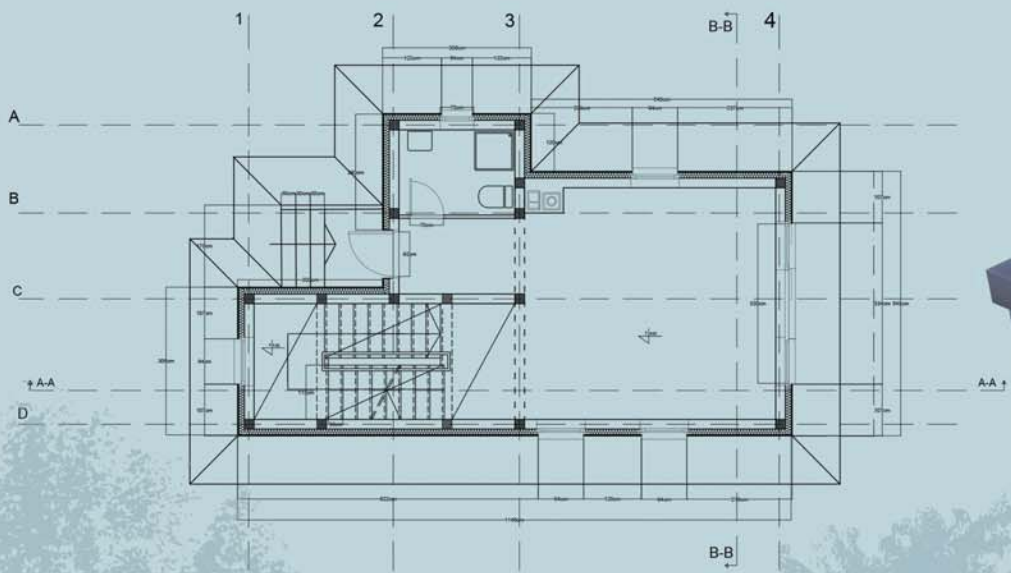
Основа приземља
