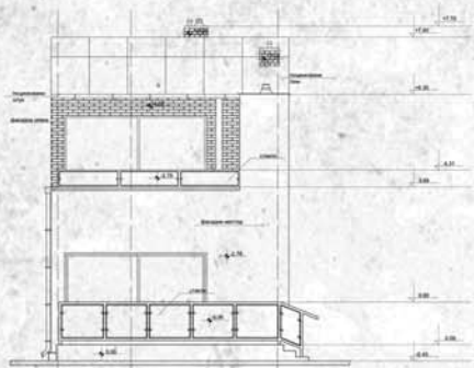
ЗАДЊИ ИЗГЛЕД
