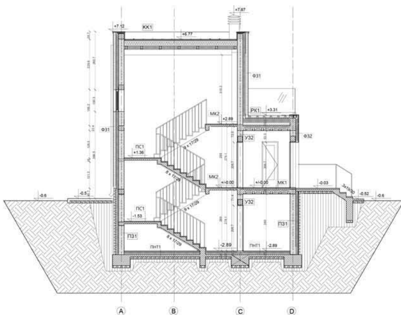
ПРЕСЕК А-А
