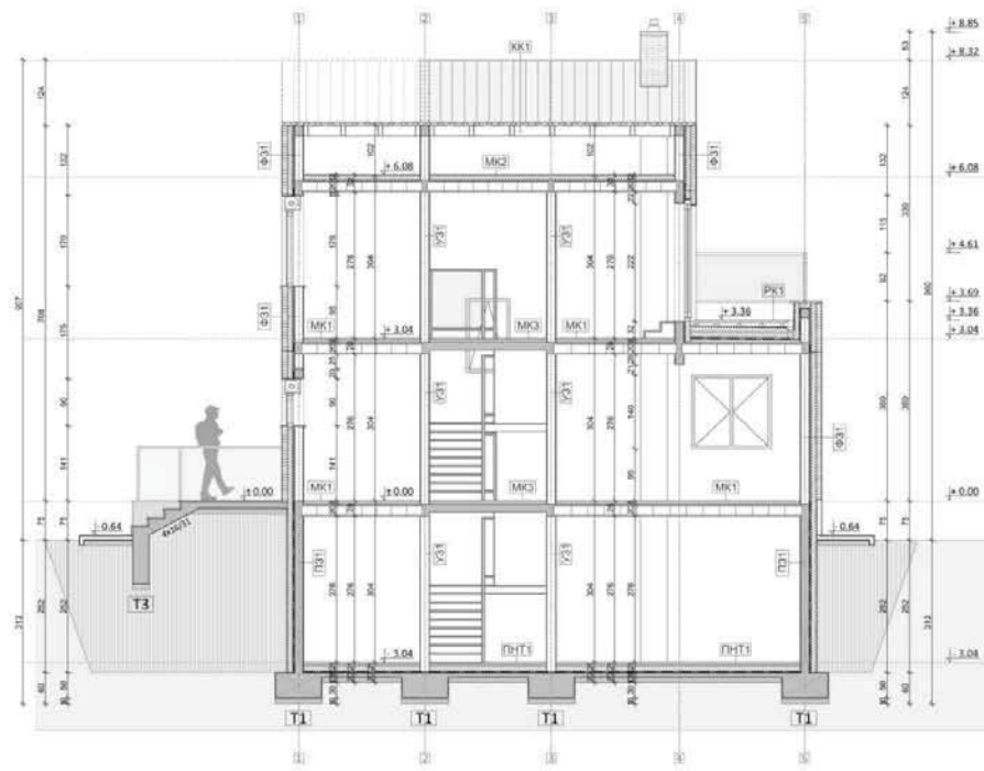
ПОДУЖНИ ПРЕСЕК
