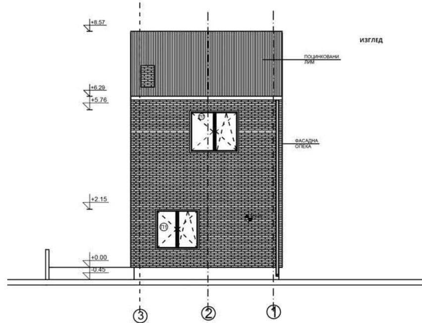
ИЗГЛЕД
