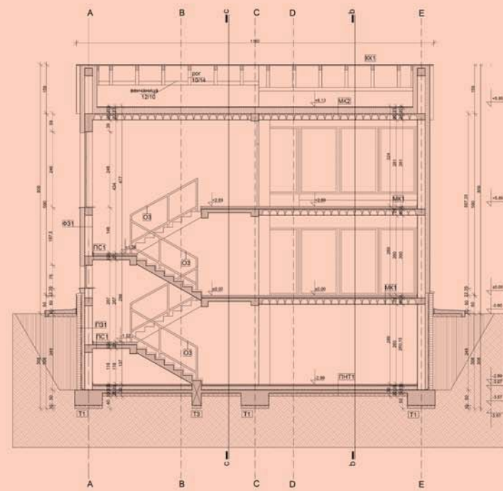
PRESEK A-A
