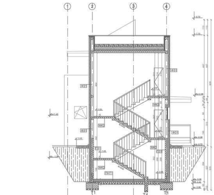
ПРЕСЕК А-А
