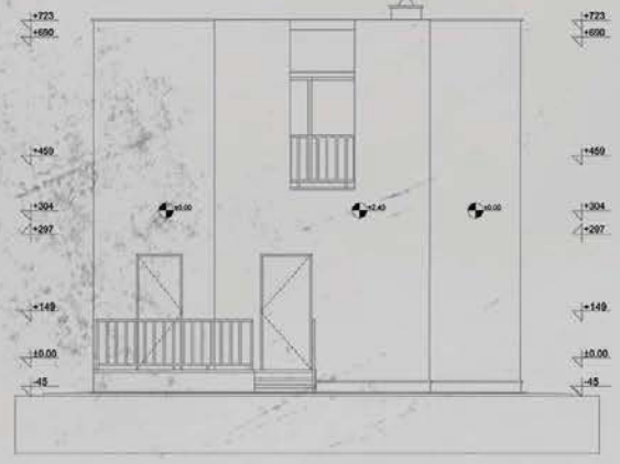
Предњи изглед
