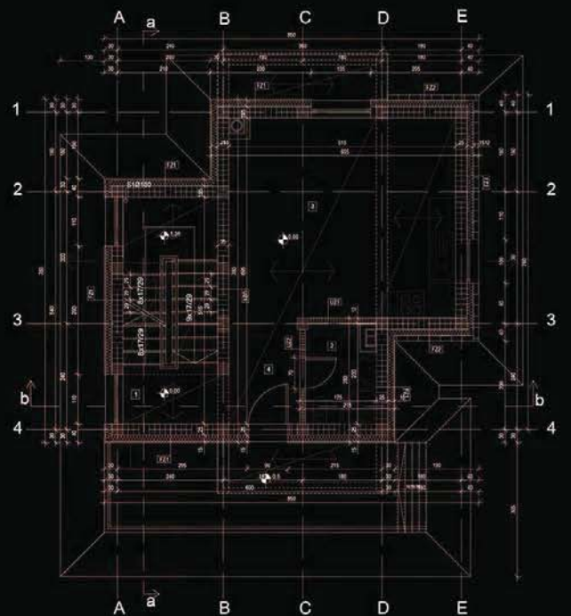
ОСНОВА СПРАТА
