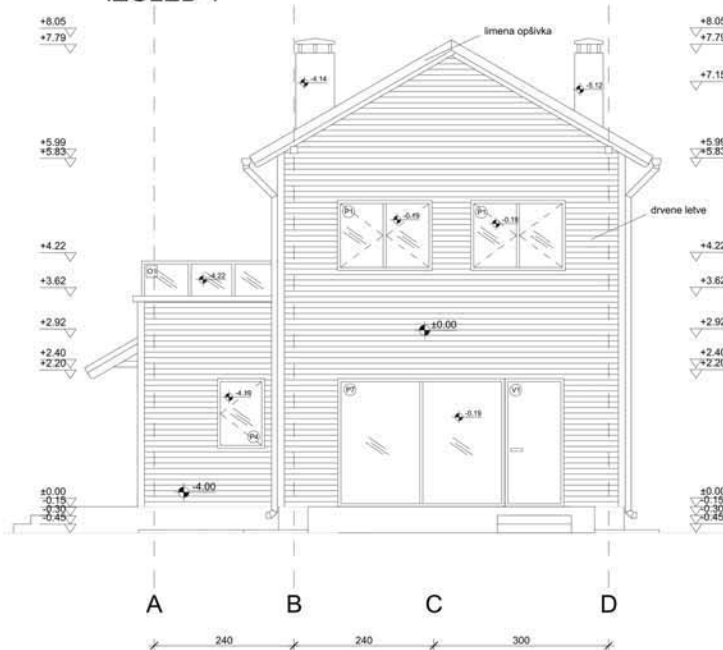
IZGLED 1
