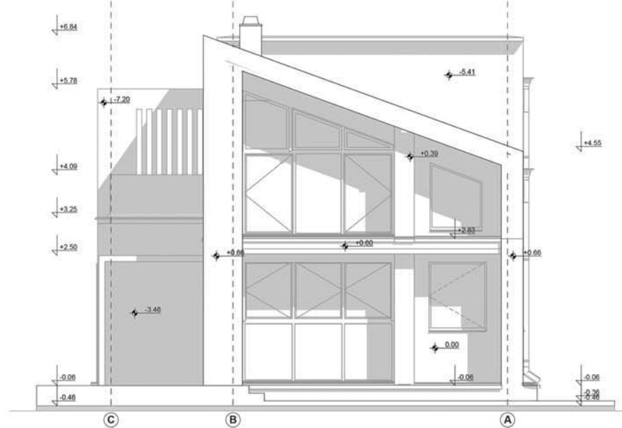
ИЗГЛЕД 3
