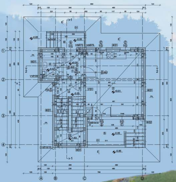
ОСНОВА ПРИЗЕМЉА
