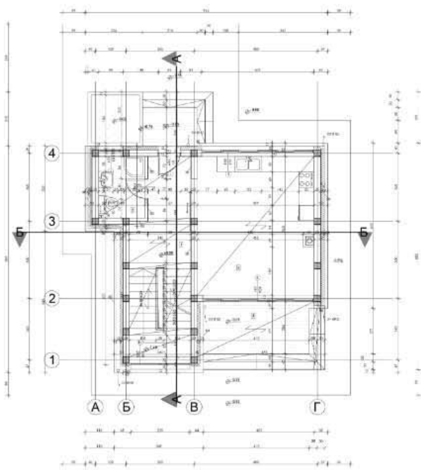
ОСНОВА ПРИЗЕМЉА
