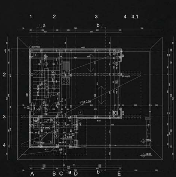
ОСНОВА ПРИЗЕМЉА
