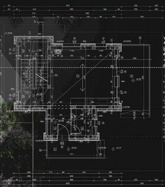
Основа приземља
