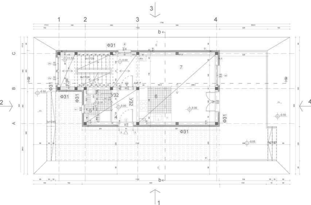
Основа приземља
