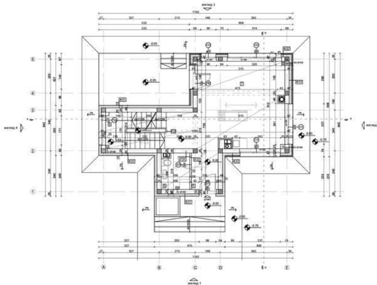
Основа приземља
