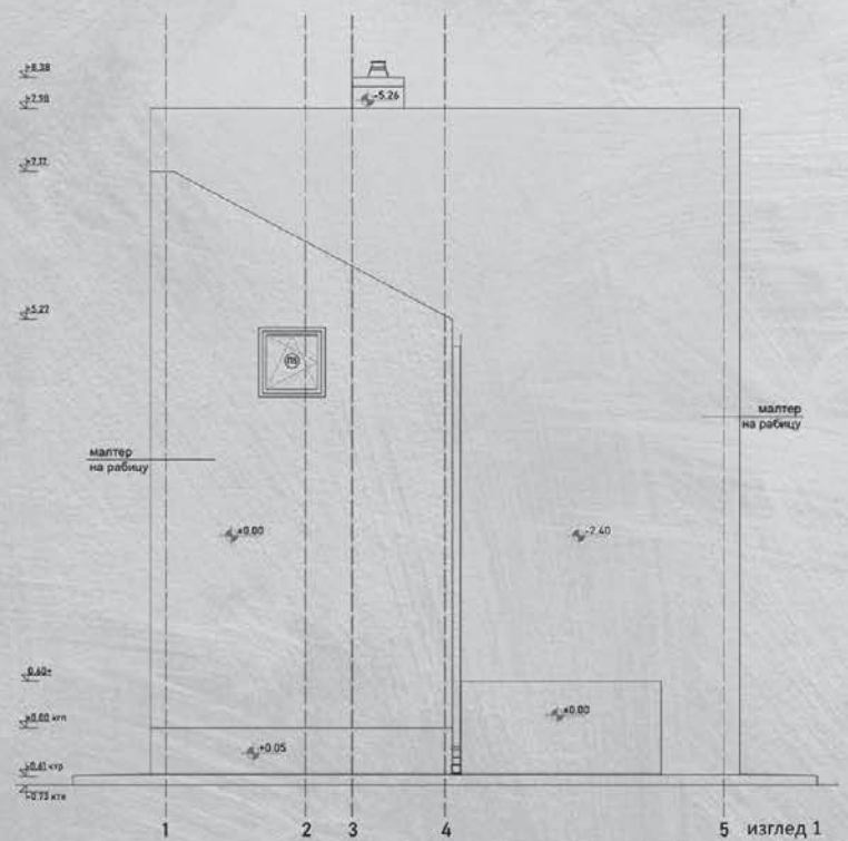
изглед 1
