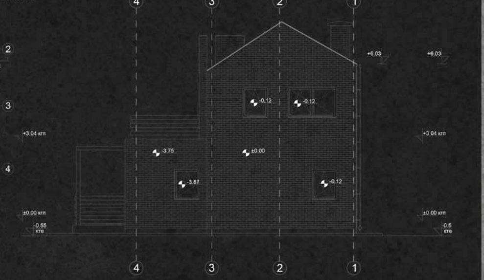
Изглед 3
