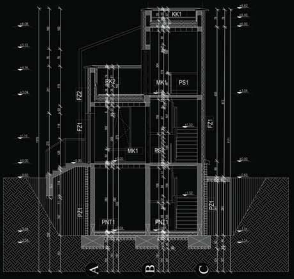
Presek B-B
