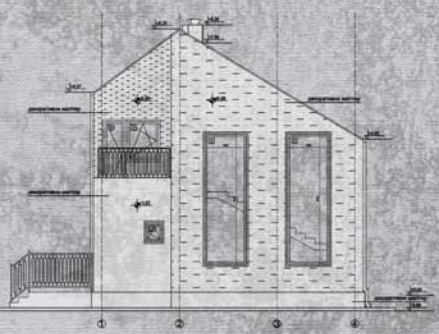
ИЗГЛЕД 1-1
