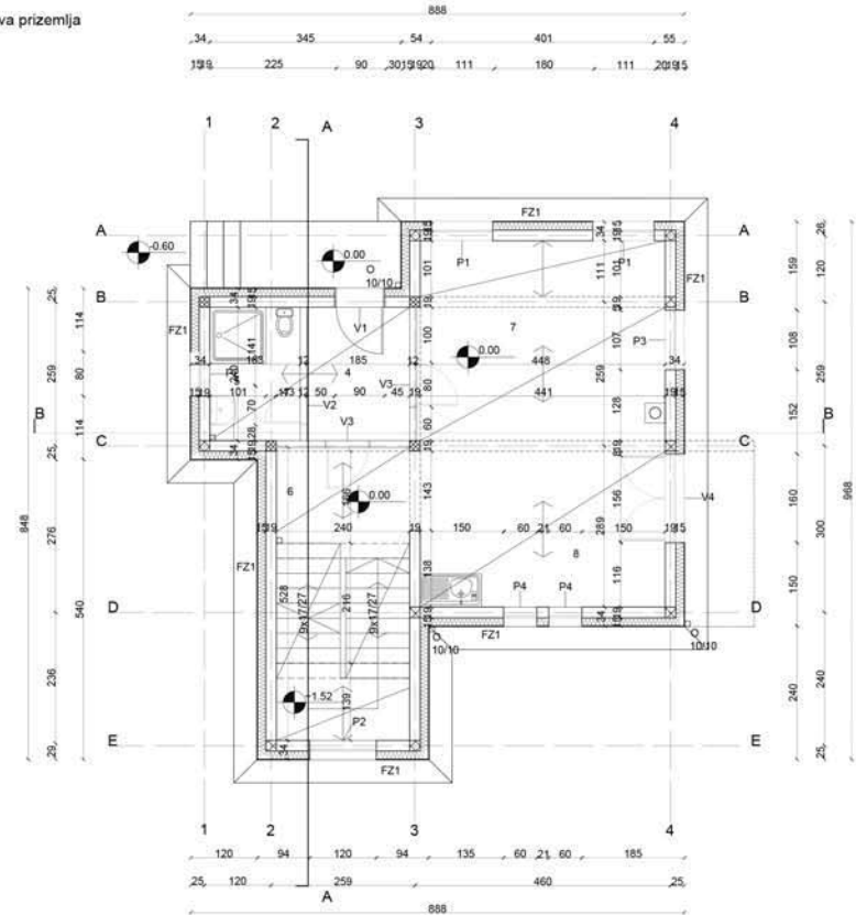
Osnova prizemlja
