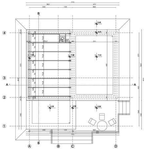
OSNOVA KROVNE KONSTRUKCIJE
