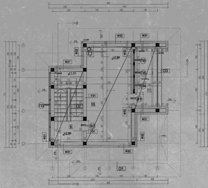
основа приземља
