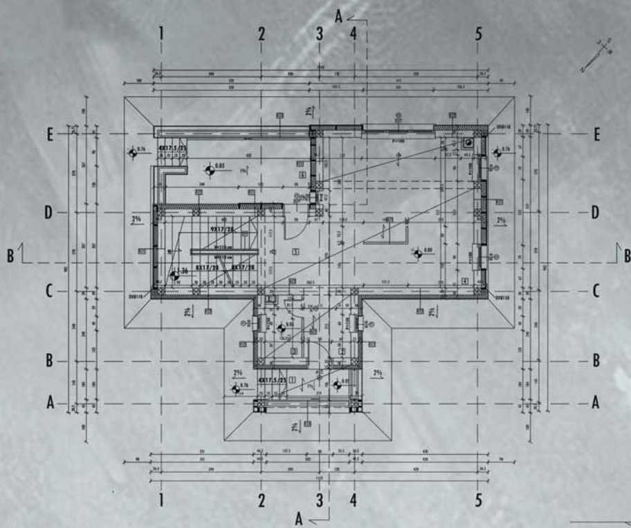
Основа приземља
