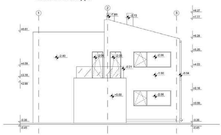
ЈУЖНА ФАСАДА
