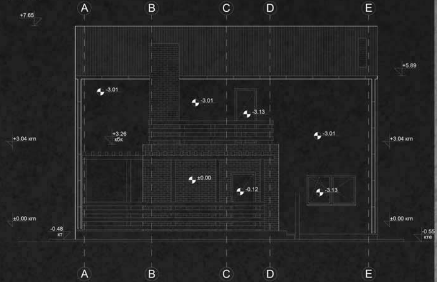
Изглед 2
