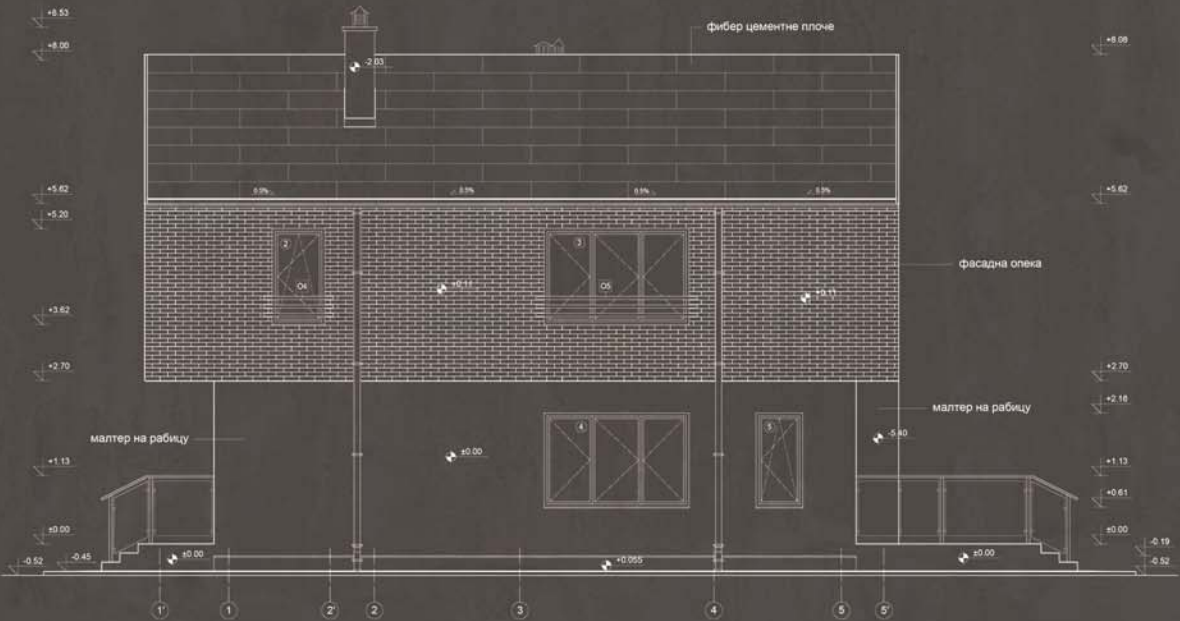
изглед
