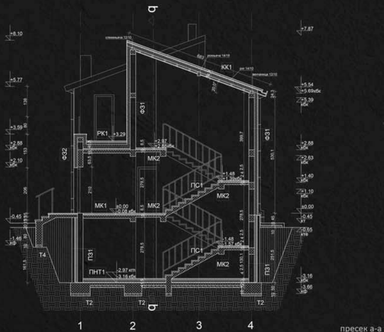
пресек а-а
