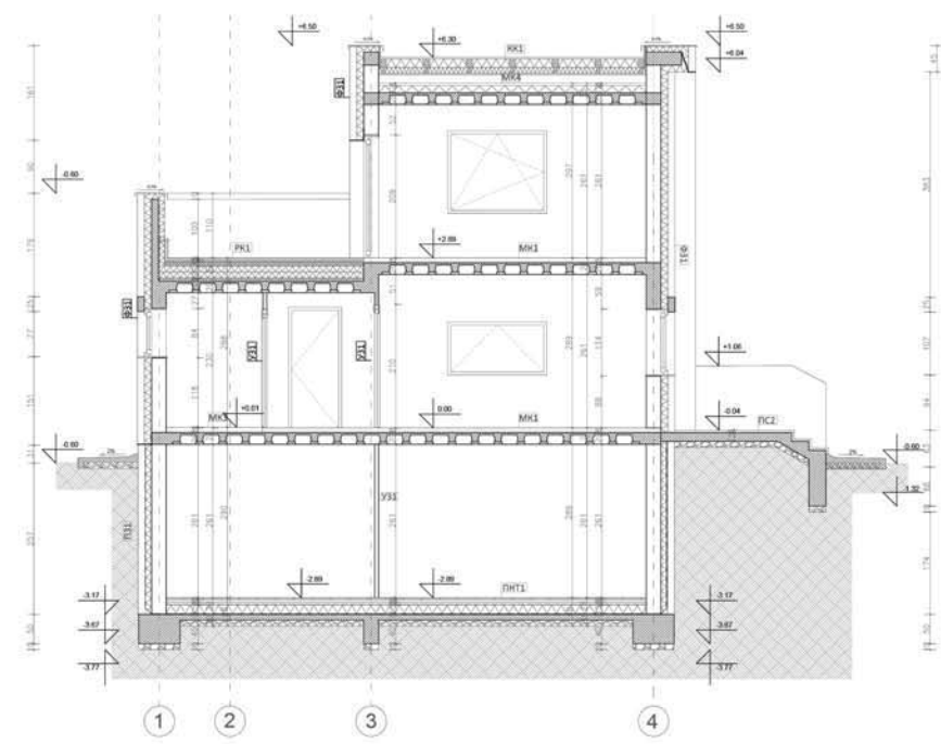
пресек 1-1
