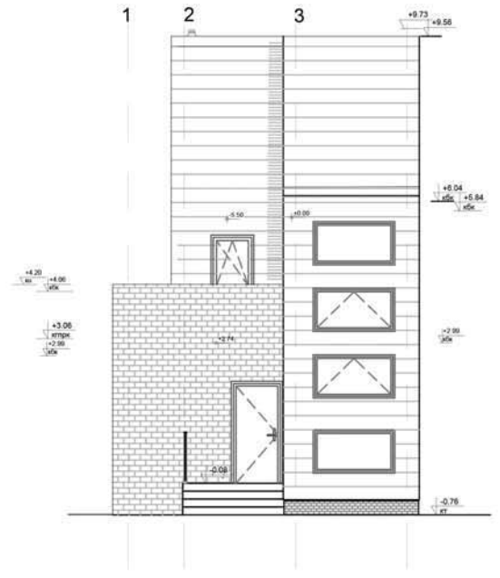
Изглед, фасада 1
