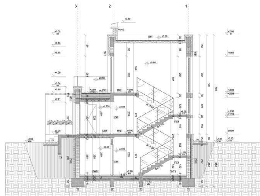
ПОДУЖНИ ПРЕСЕК 6-6
