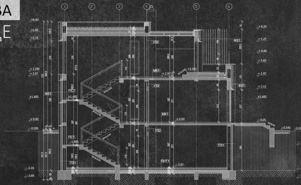
///Подужни пресек
