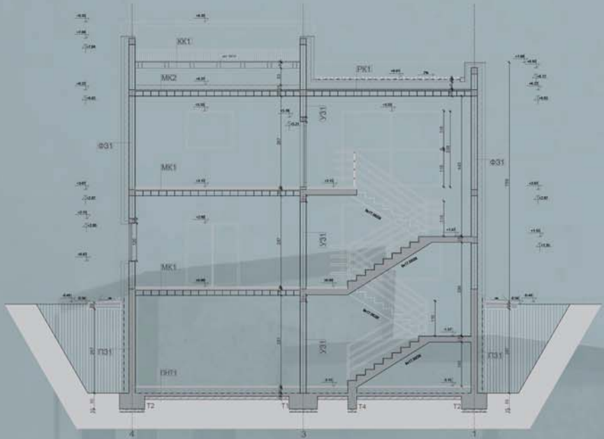
пресек b-b
