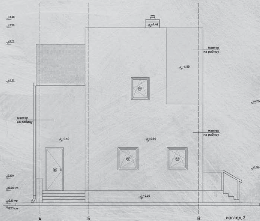
изглед 2
