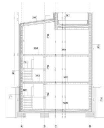
PRESEK a-a
