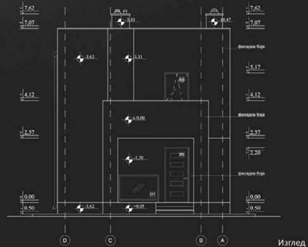
Изглед
