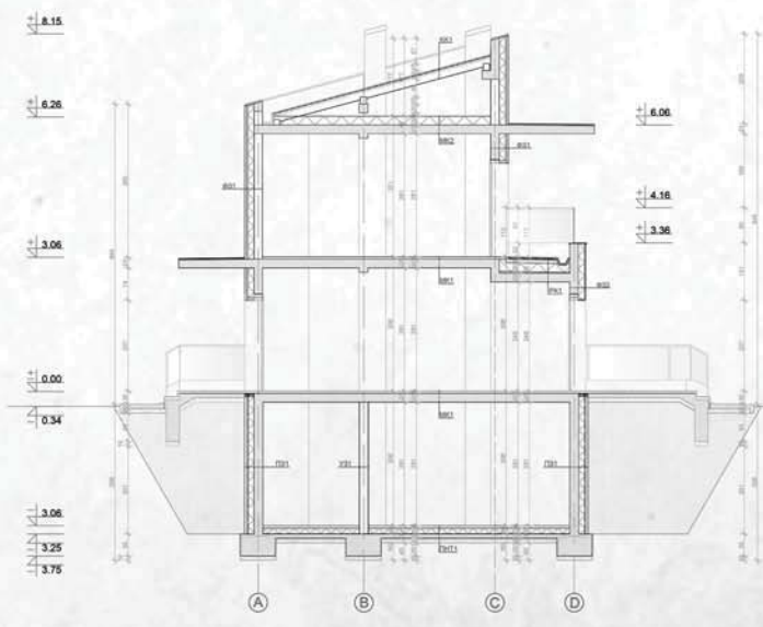
пресек С-С
