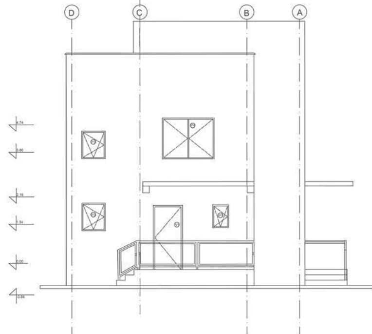
ИЗГЛЕД 2
