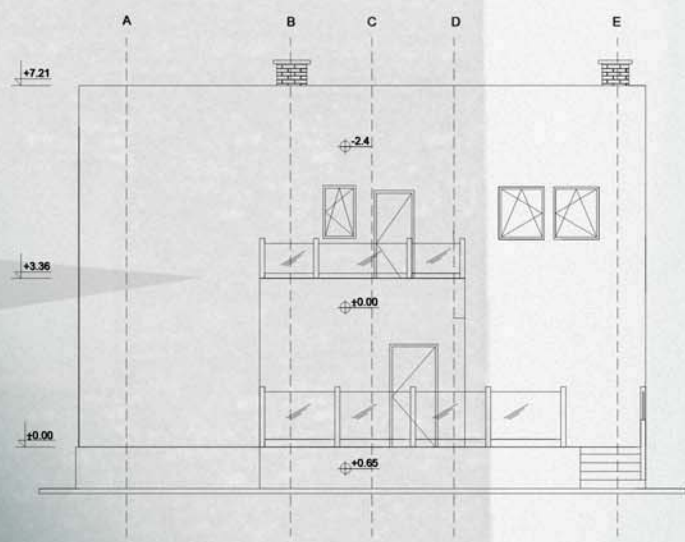
ИЗГЛЕД 1
