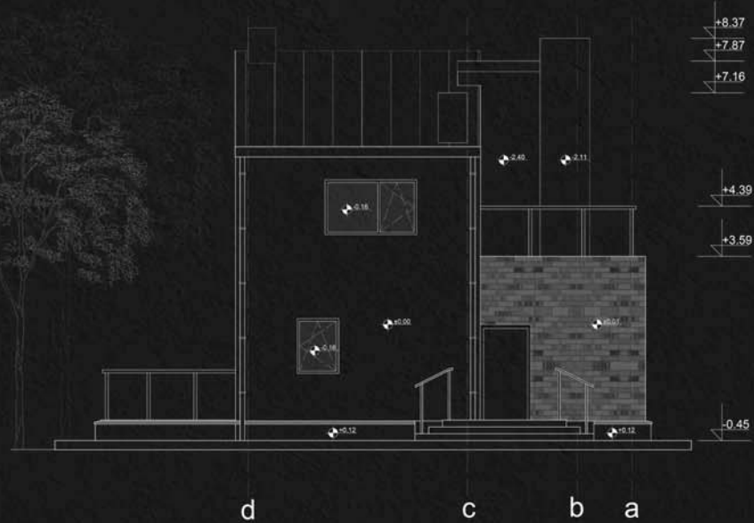
изглед 1
