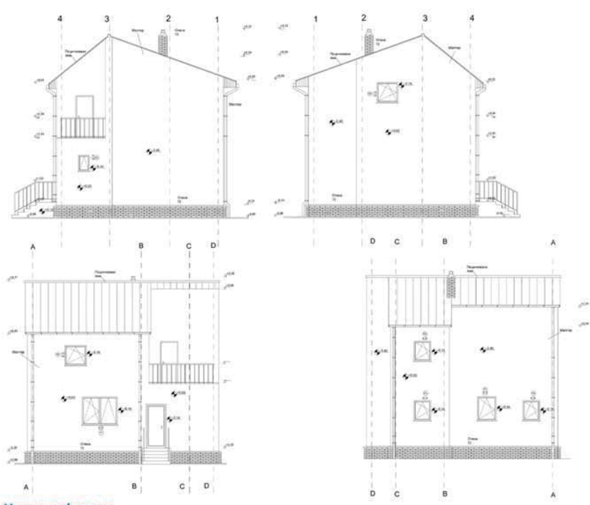
Изгледи фасаде
