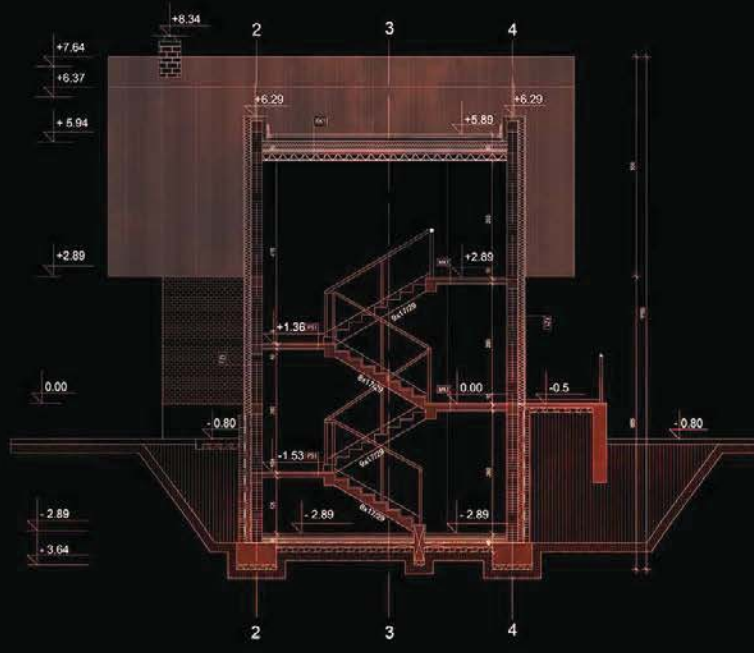
ПРЕСЕК а-а
