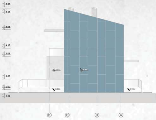
изглед 1
