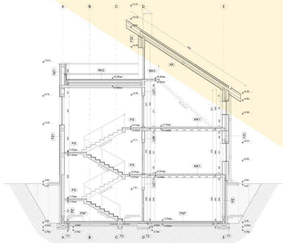
Presek A-A
