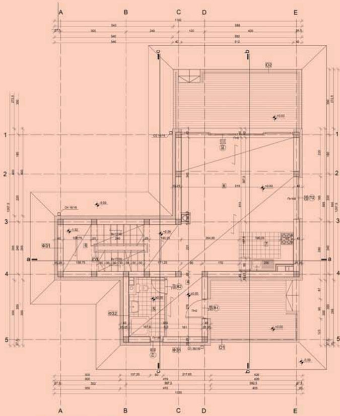
OSNOVA PRIZEMLJA
