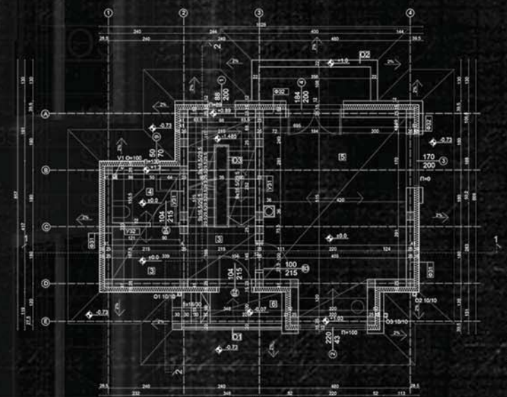
//osnova prizemlja
