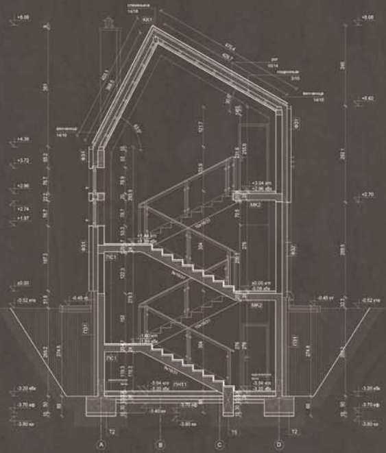
попечни пресек
