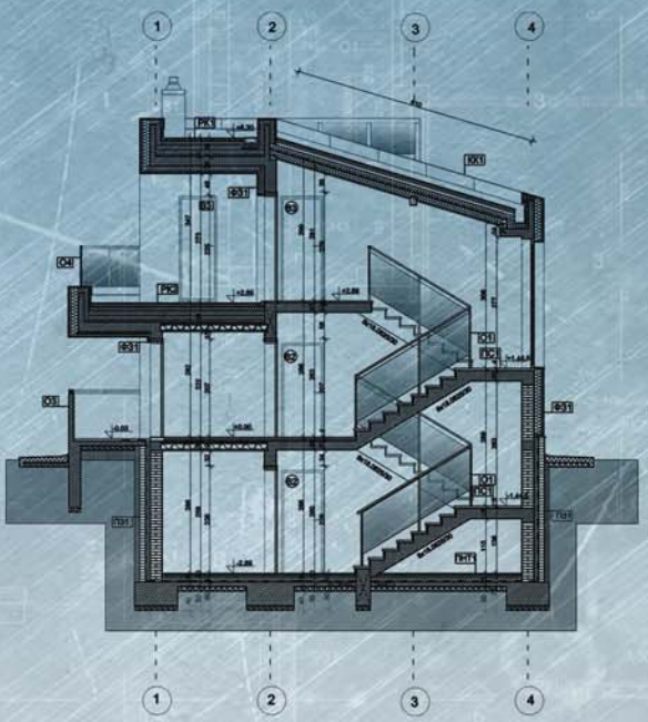
Пресек А-А
