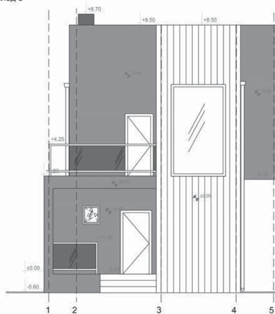
изглед 3
