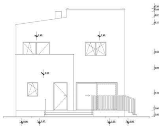
IZGLED - LICE
