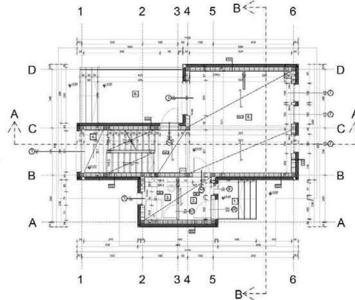
ОСНОВА ПРИЗЕМЉА 1:50
