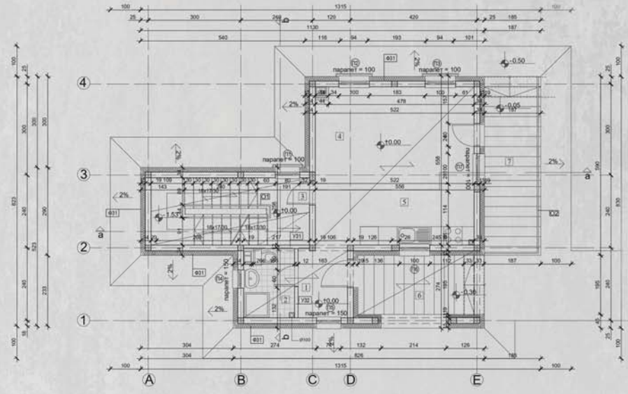
Основа приземља
