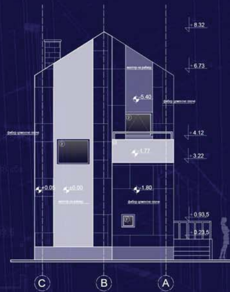
изглед
