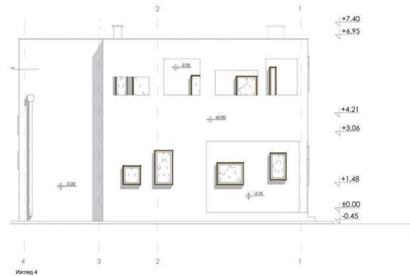
Изглед 4
