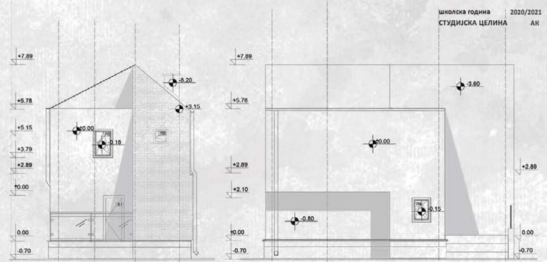
Изглед 2
