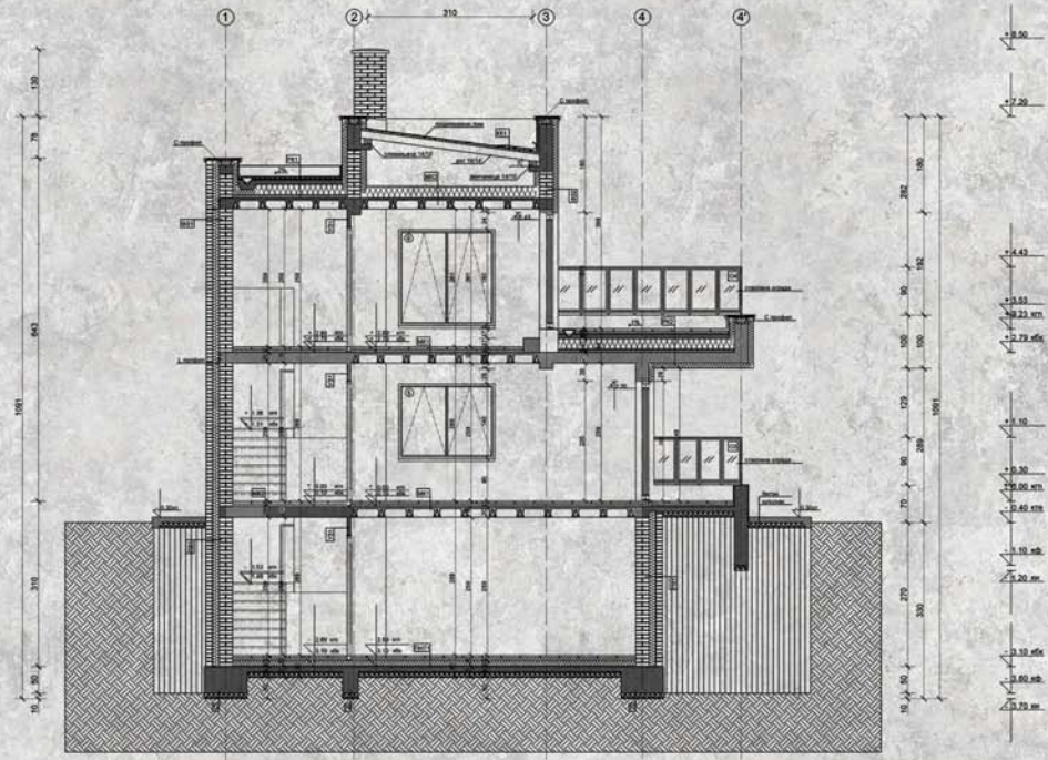
пресек АА
