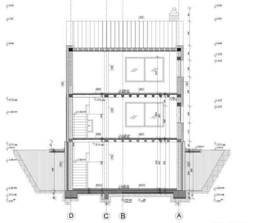
ПРЕСЕК а-а
