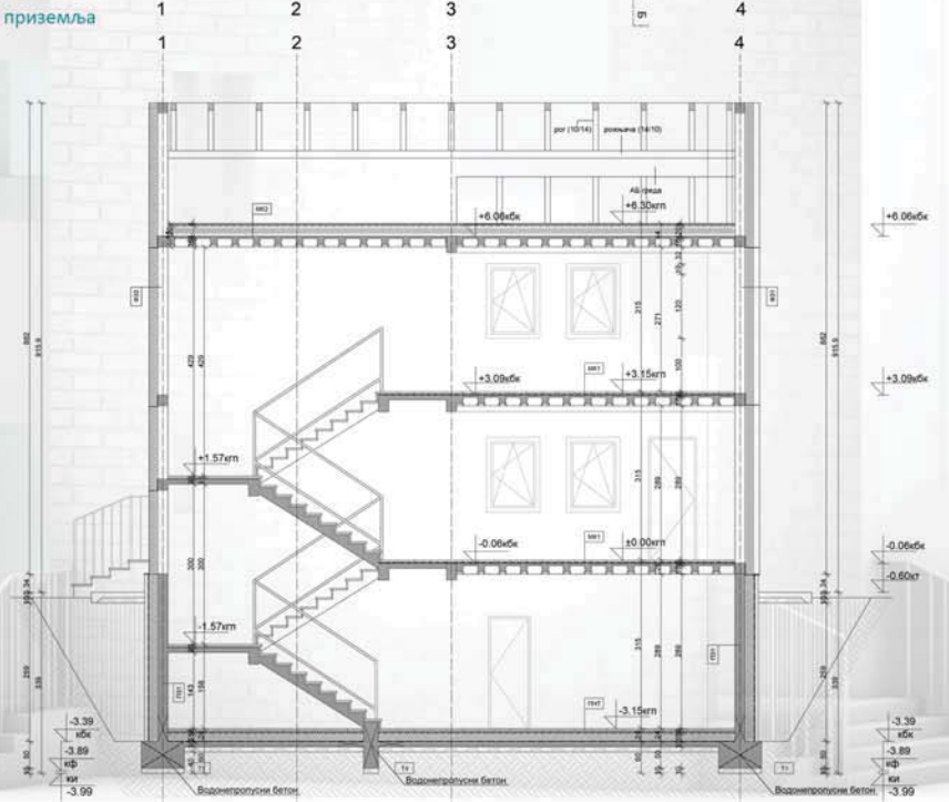
Подужни пресек
