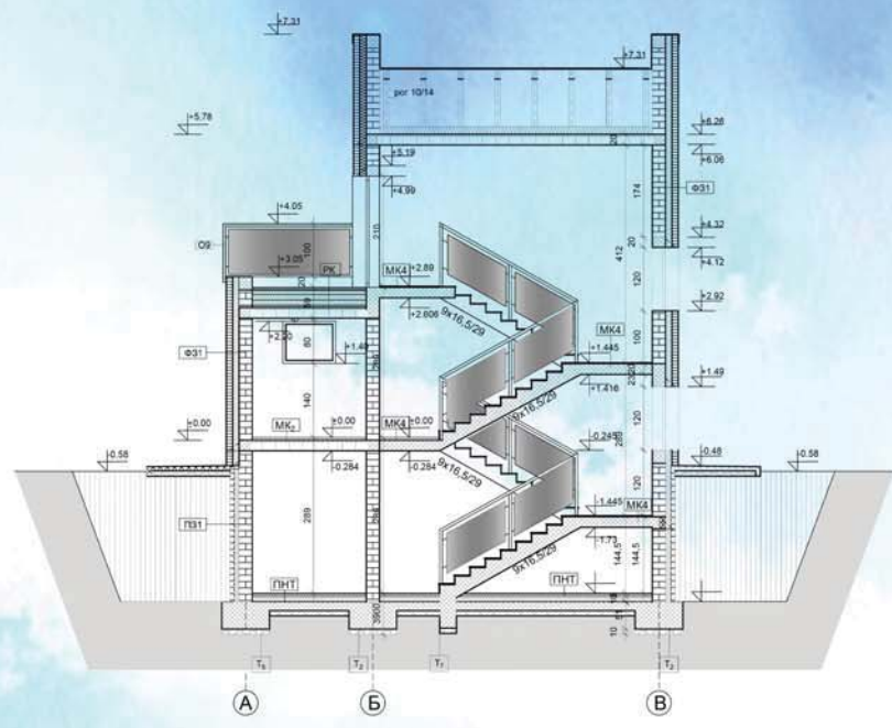
ИЗГЛЕД 1
