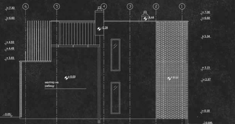
///Изглед
