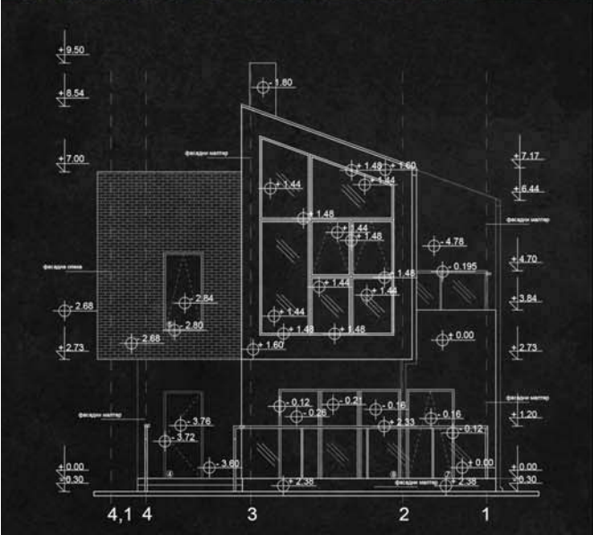
ИЗГЛЕД
