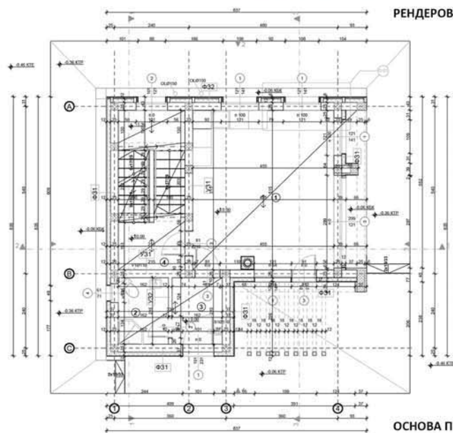
ОСНОВА ПРИЗЕМЉА
