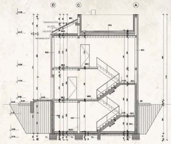
Пресек А-А
