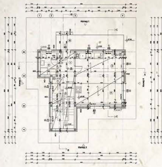
Основа приземља
