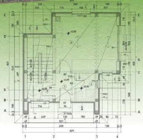
основа приземља
