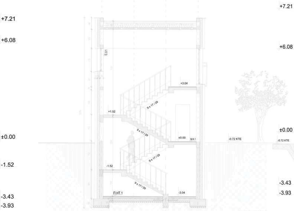
пресек Б - Б
