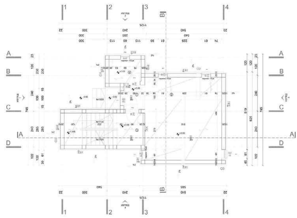
ОСНОВА ПРИЗЕМЉА
