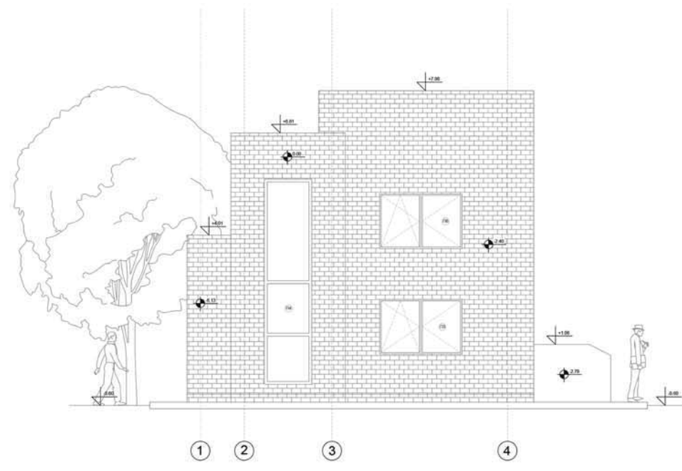
изглед
