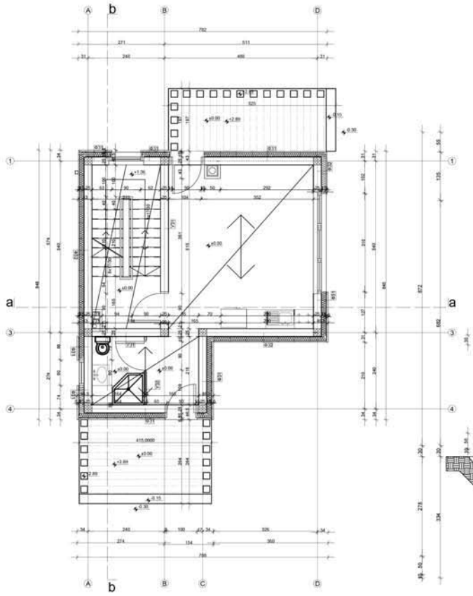
Основа приземља
