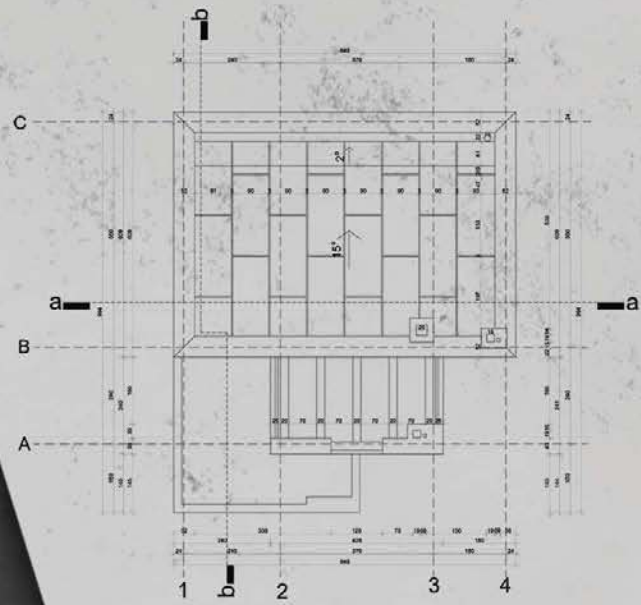
Основа крова
