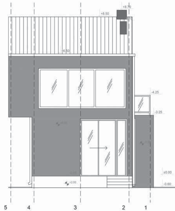
изглед 1
