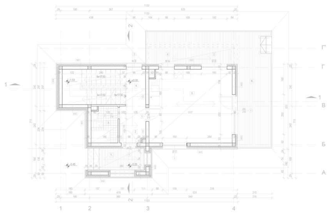
основа приземља
