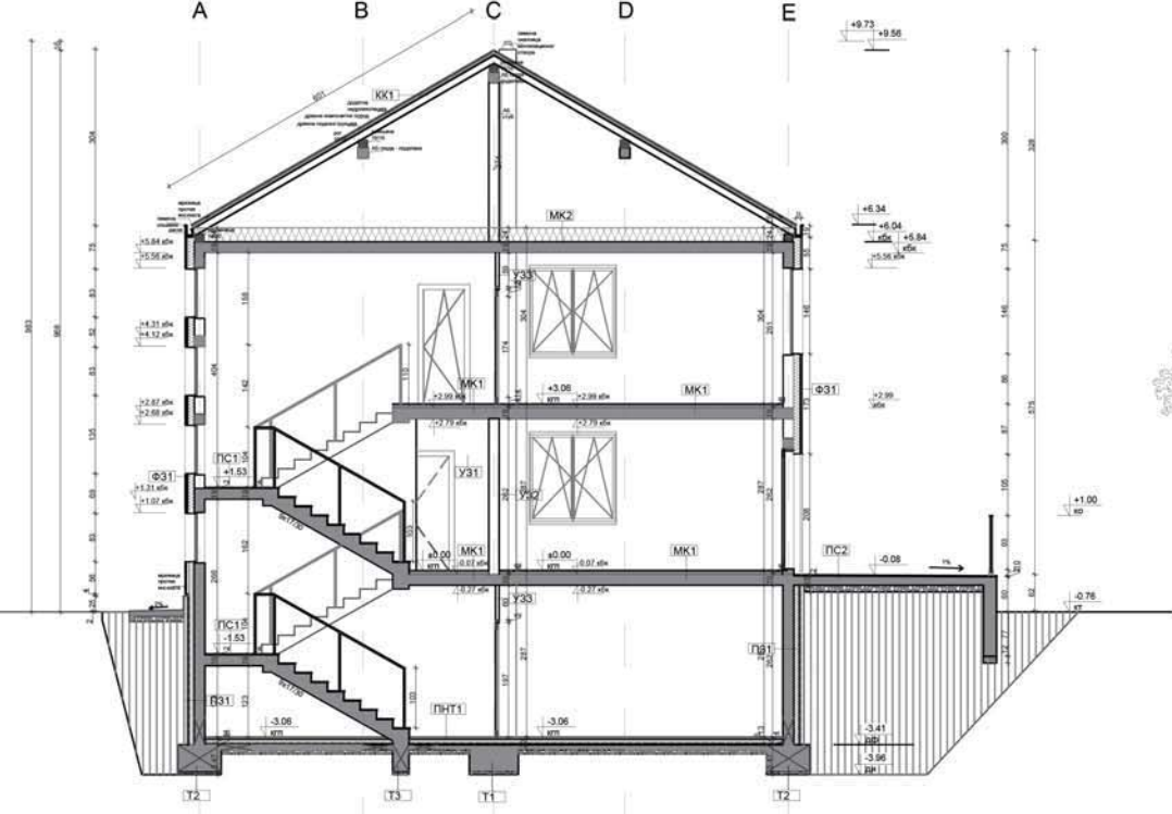
Пресек а-а
