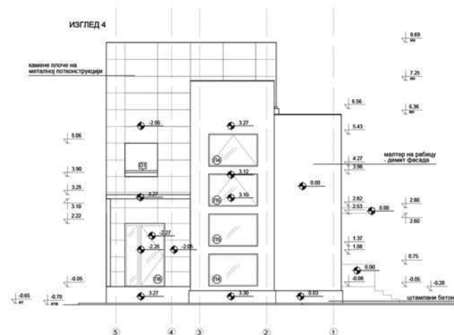
Изглед 4
