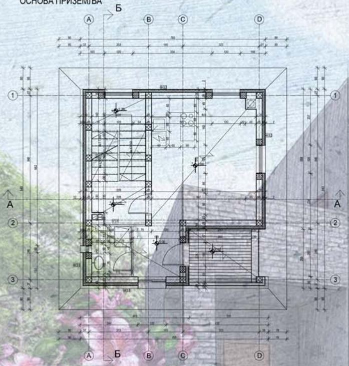
ОСНОВА ПРИЗЕМЉА
