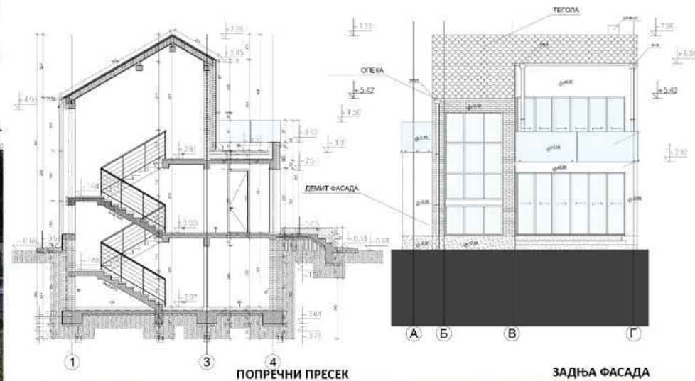
ПОПРЕЧНИ ПРЕСЕК
