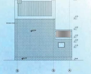
ИЗГЛЕД 4
