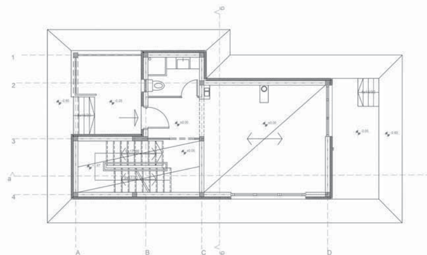
основа приземља
