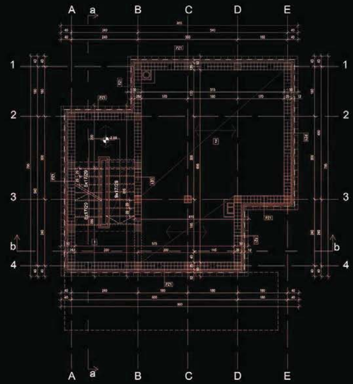
ОСНОВА ПОДРУМА
