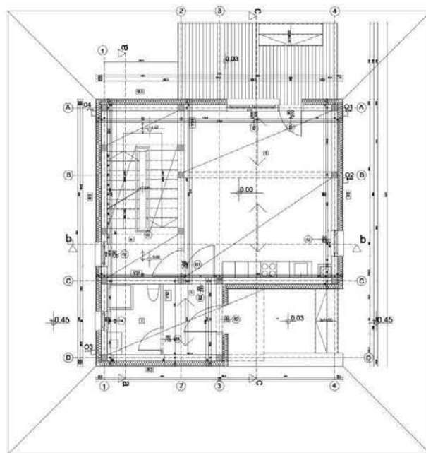
ОСНОВА ПРИЗЕМЉА
