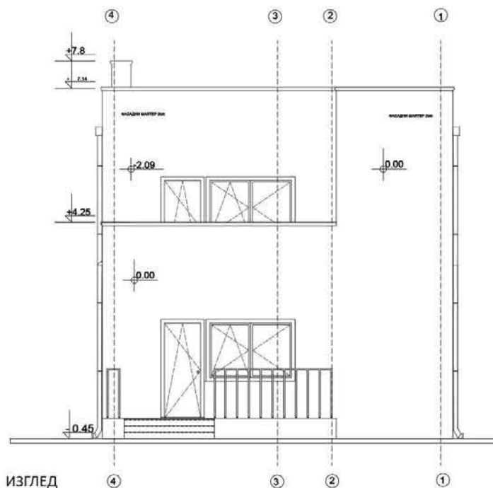
ИЗГЛЕД
