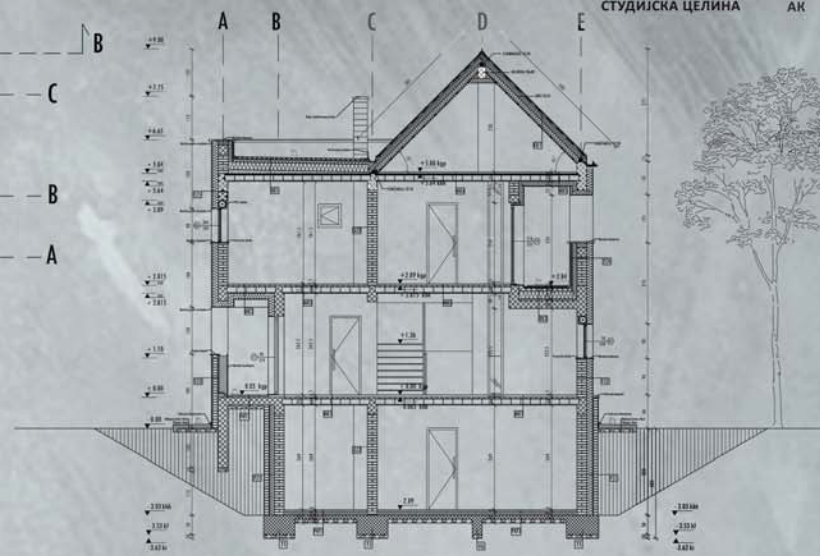
Пресјек А-А
