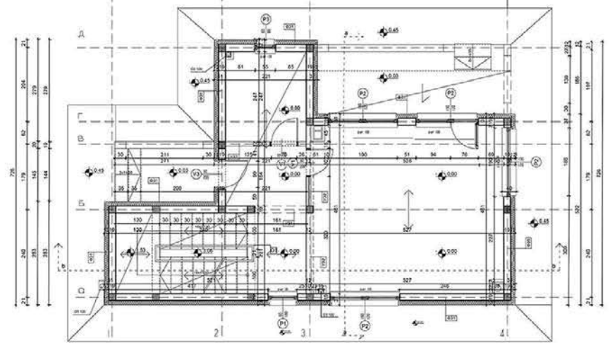
Основа приземља
