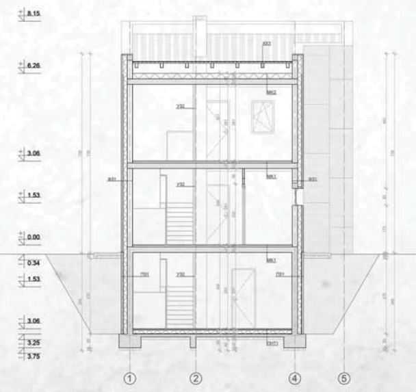
пресек В-В
