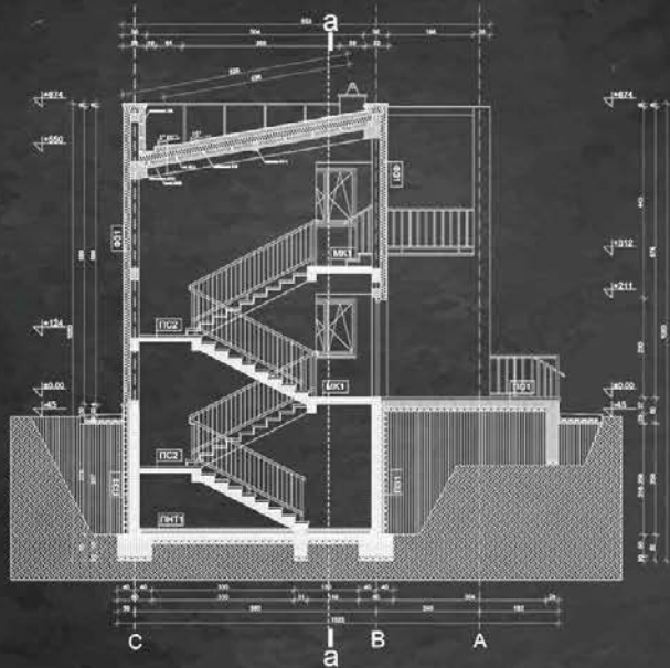
Попречни пресек
