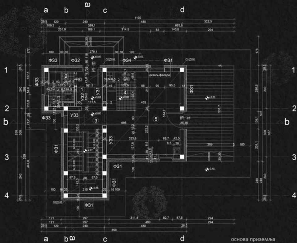
основа приземља
