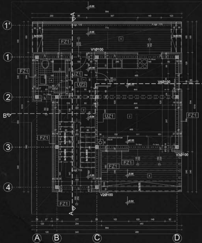
ОСНОВА ПРИЗЕМЉА
