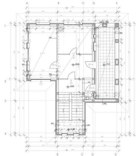
Изглед 2
