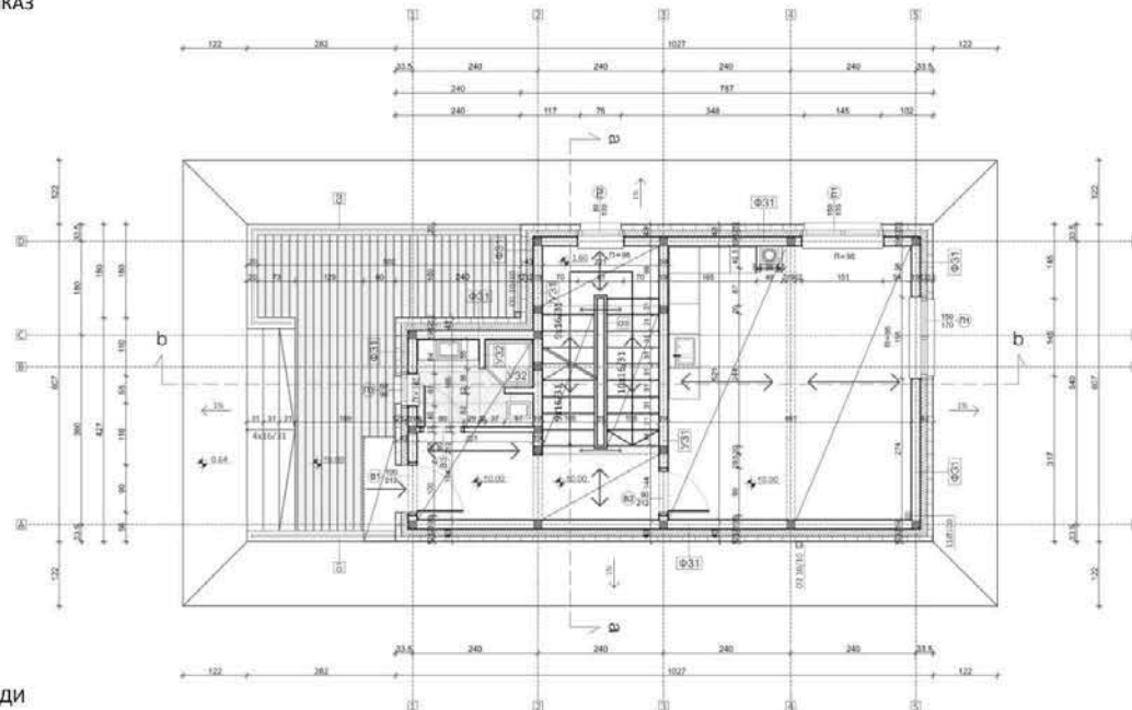
ОСНОВА ПРИЗЕМЉА
