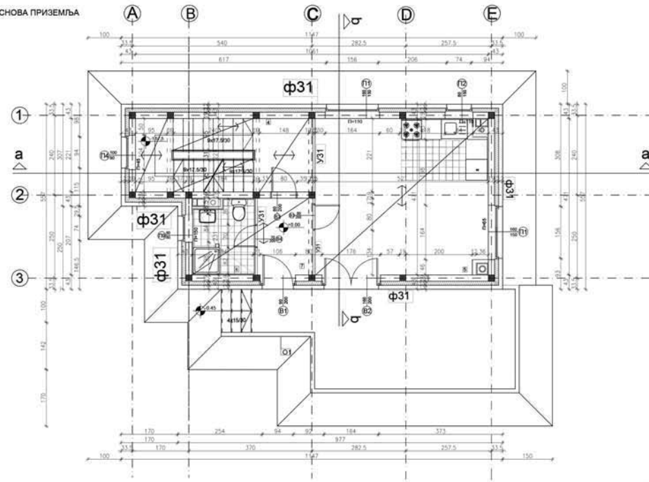
ОСНОВА ПРИЗЕМЉА
