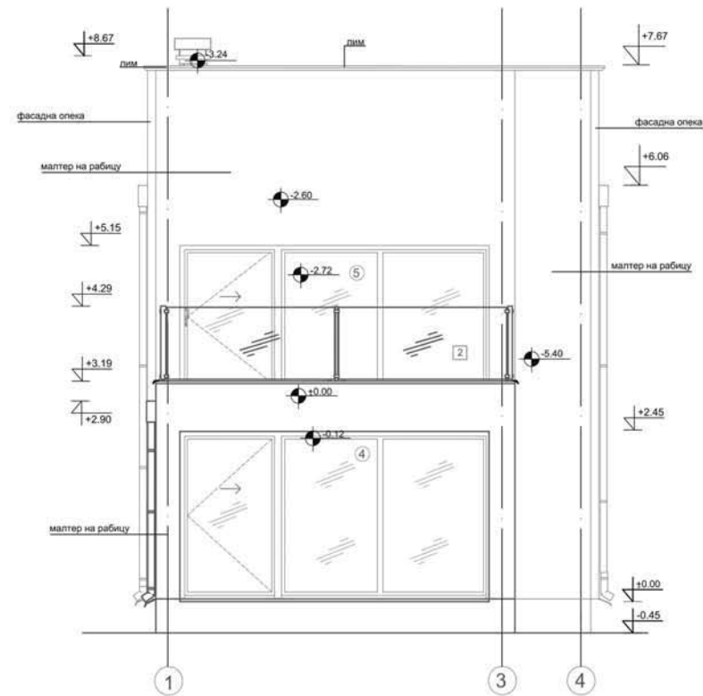
ИЗГЛЕД- ЛИЦЕ
