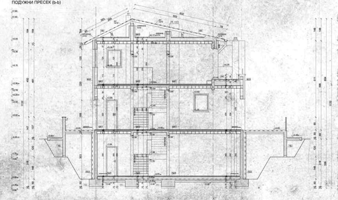
ПОДУЖНИ ПРЕСЕК (b-b)
