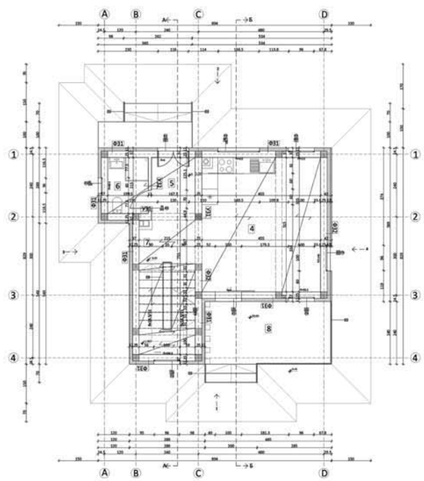
ОСНОВА ПРИЗЕМЉА
