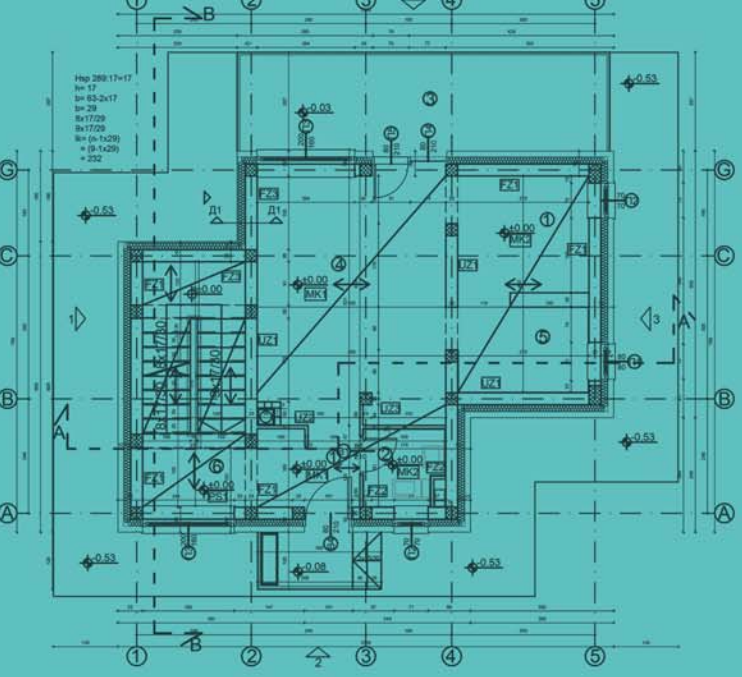
Основа приземља R 1:50
