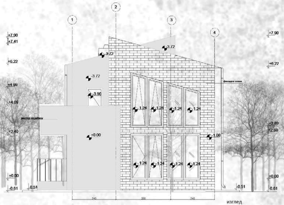
изглед
