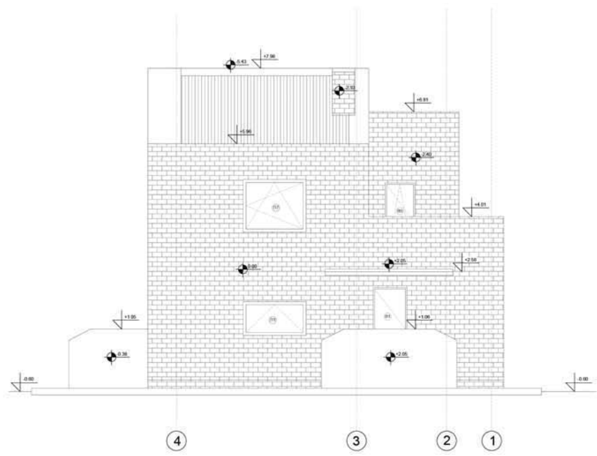
изглед
