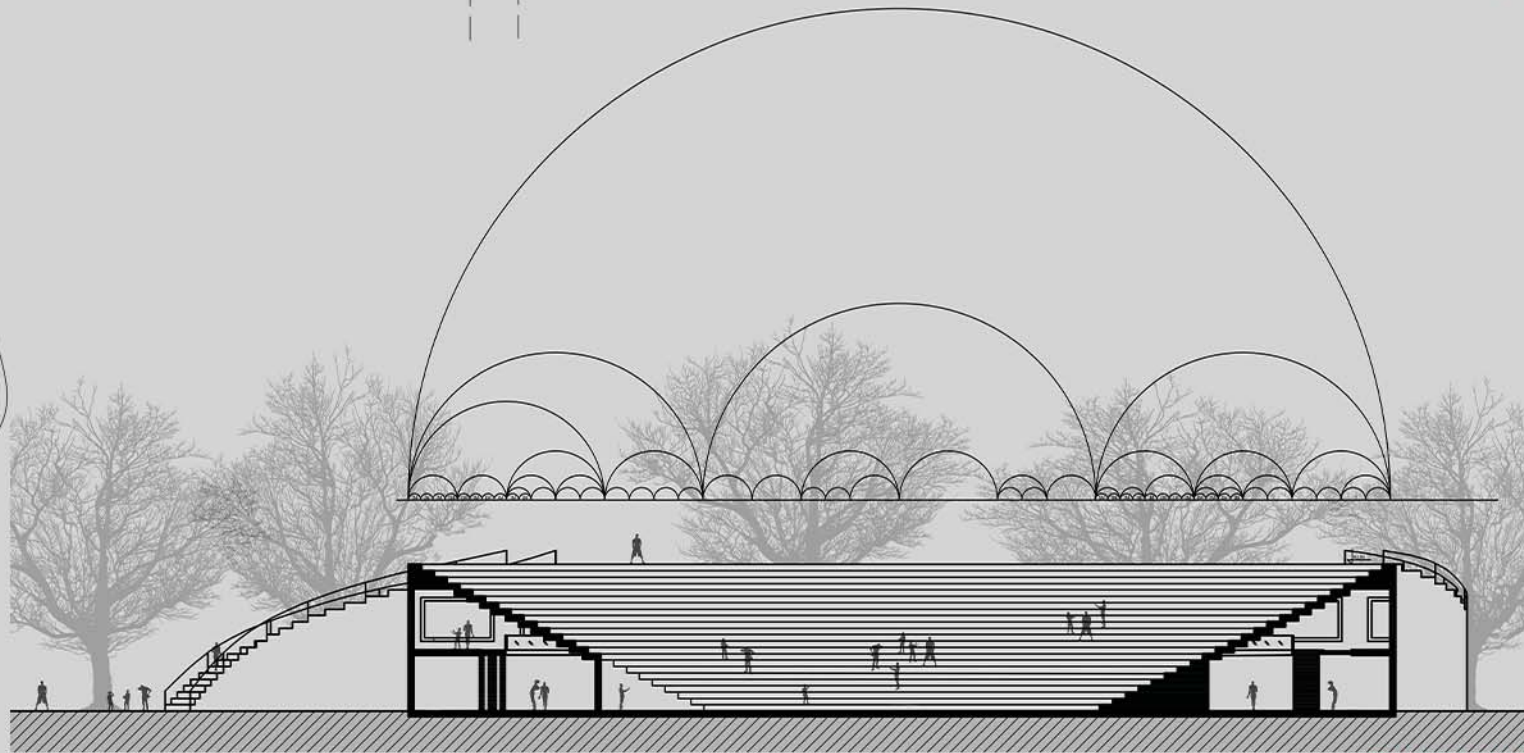
ПРЕСЕК ПАВИЉОНА БР.1
