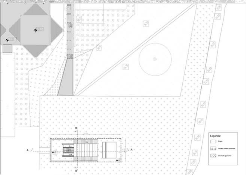
Ситуација Р=1:200
