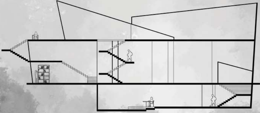
PRESEK A-A
