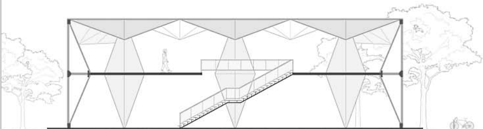
Подужни пресек
