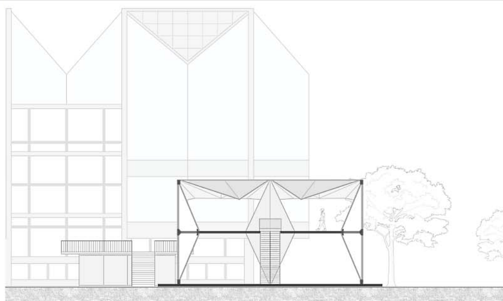
Попречни пресек
