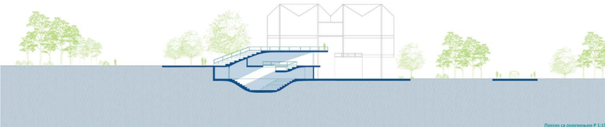
Пресек са окружењем Р 1:150
