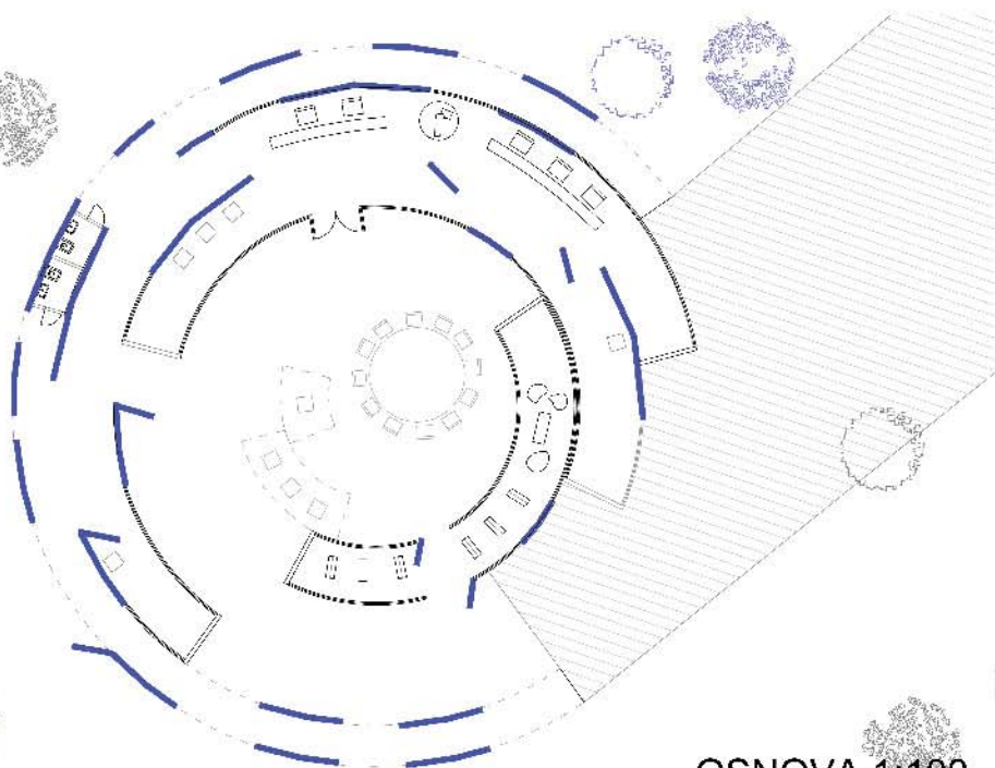
OSNOVA 1:100
