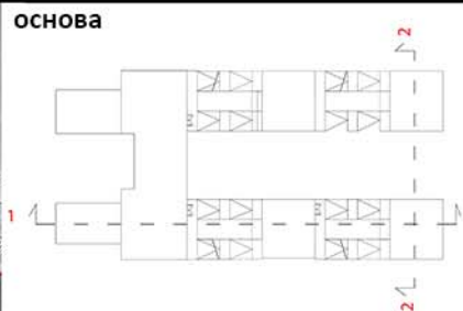
основа
