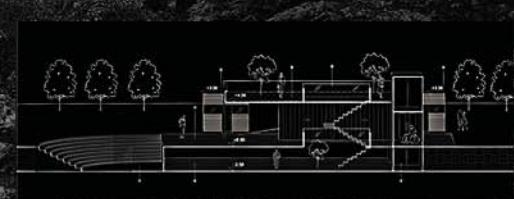
подужни пресек- кроз амфитеатар
