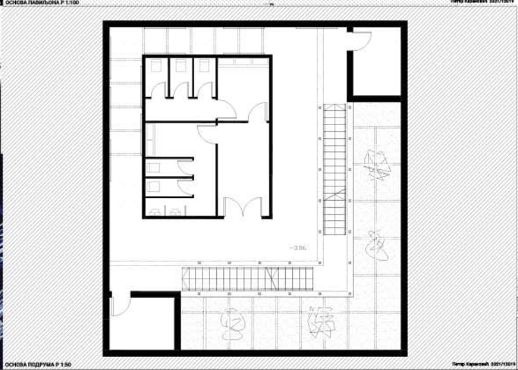
ОСНОВА ПОДРУМА Р 1:50
