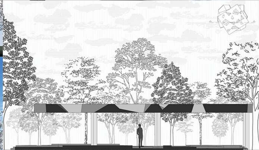
Dragana Kukobat 2021/11233 Пресек R 1:50
