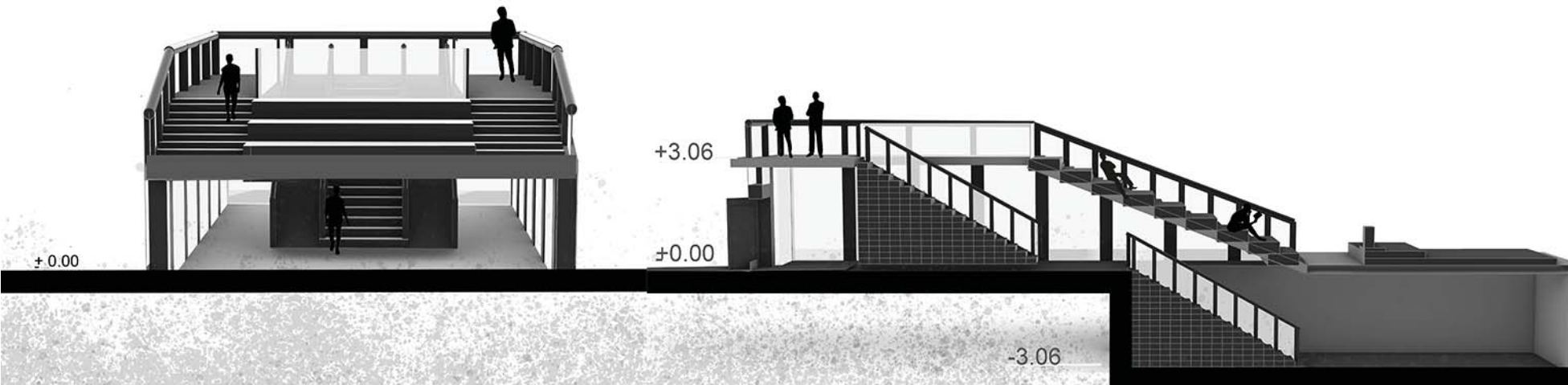
Пресек Б-Б
