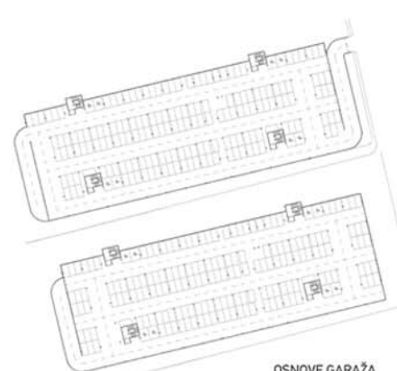
OSNOVE GARAŽA R = 1:500
