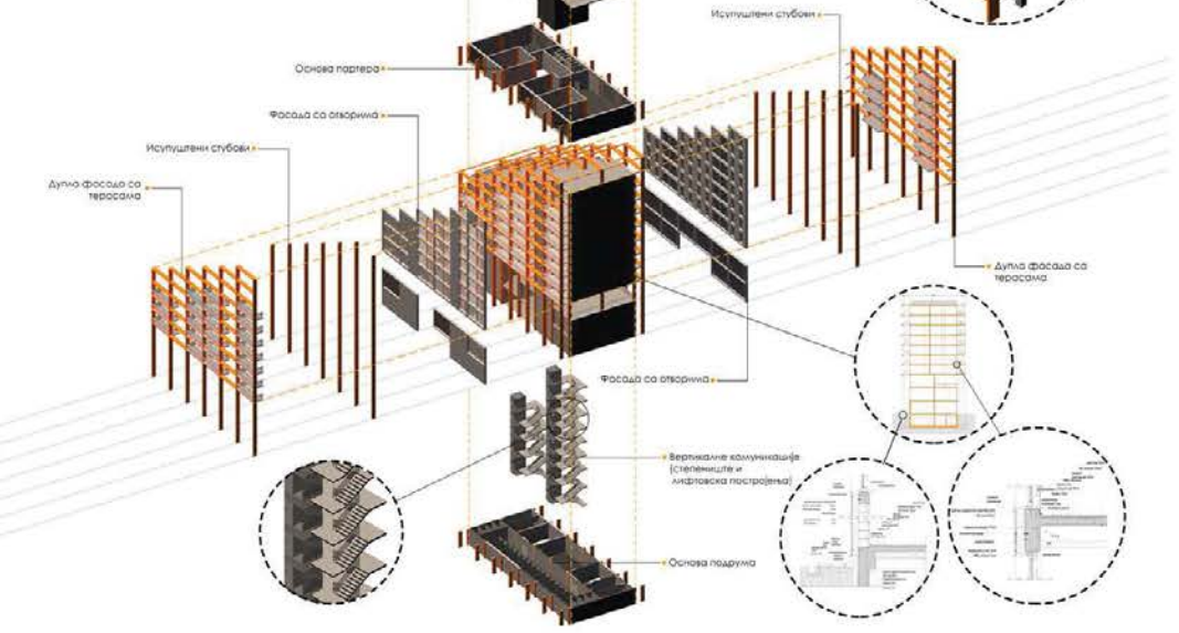
ЕКСПЛОДИРАНА АКСОНОМЕТРИЈА
