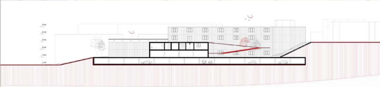
попречни пресек
