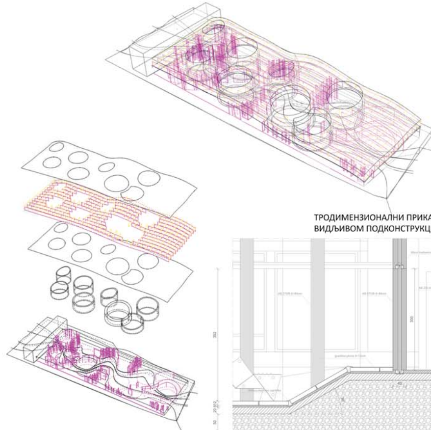
ЕКСПЛОДИРАНИ ПРИКАЗ СЛОЈЕВА КОНСТРУКЦИЈЕ
