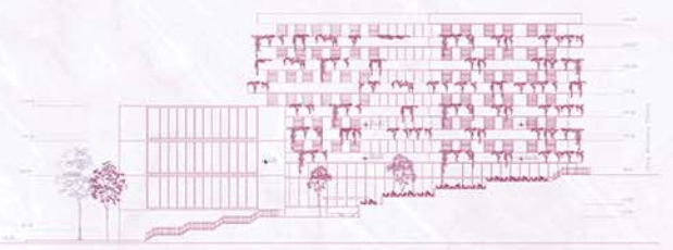
Izgled 1 R 1:250
