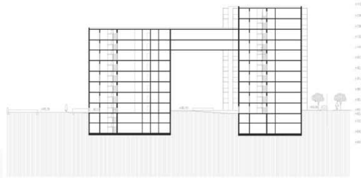
PRESEK 3-3b 1:250
