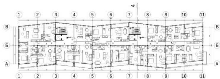
основа спрата стамбеног објекта на коти +3.20
