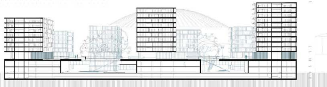
Пресек
