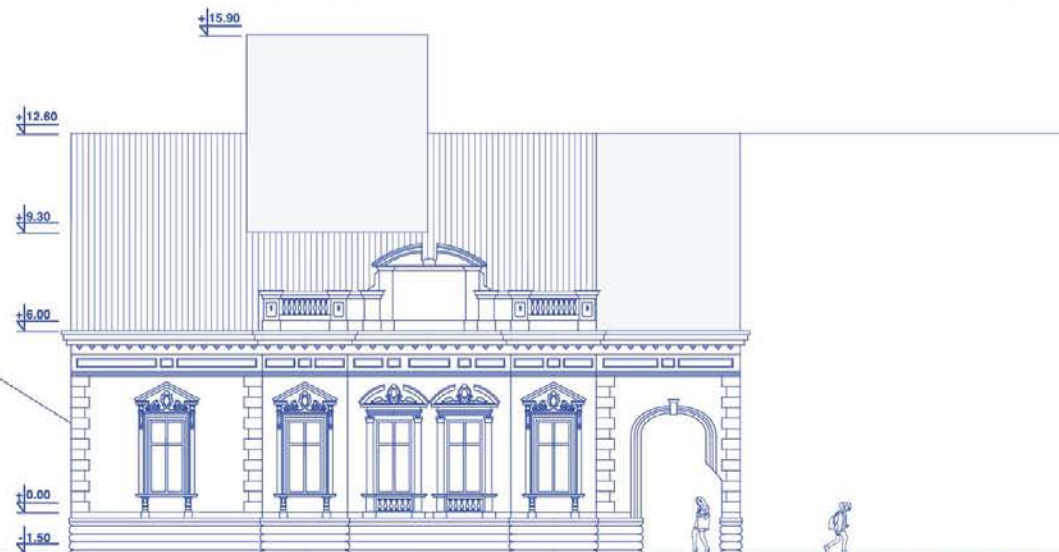
ИЗГЛЕД ГЛАВНЕ ФАСАДЕ
