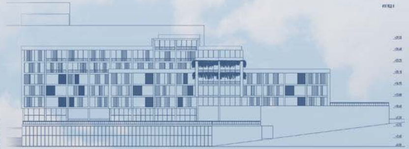
изгледи
