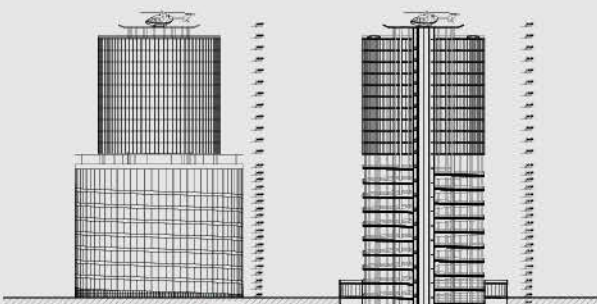
Изглед
