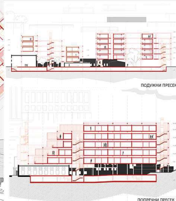
ПОПРЕЧНИ ПРЕСЕК
