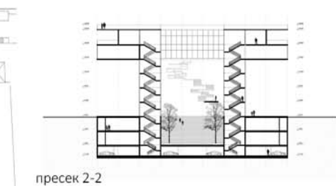
пресек 2-2
