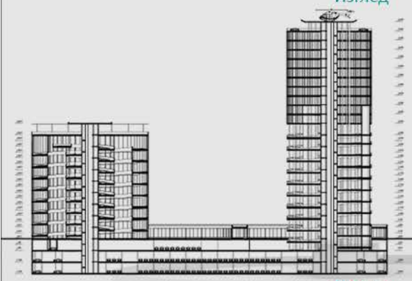
Пресек
