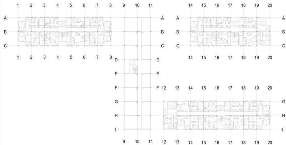
Основа
