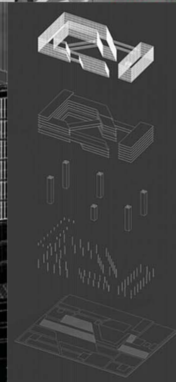
ЕКСПЛОДИРАНА АКСОНОМЕТРИЈА
