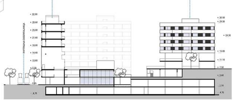
ПОПРЕЧНИ ПРЕСЕК
