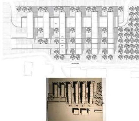
ситуационо решење
