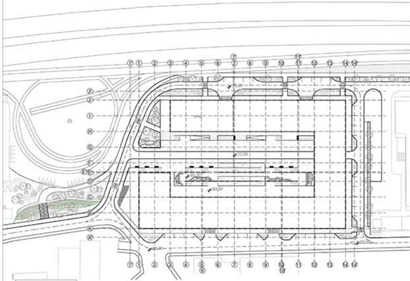
OSNOVA PRIZEMLJA R 1:100
