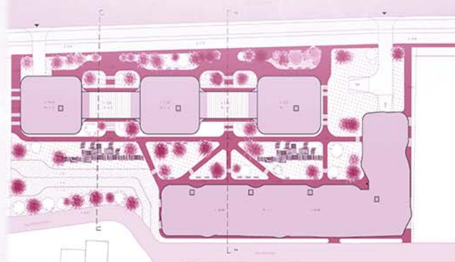
Situacija R 1:250
