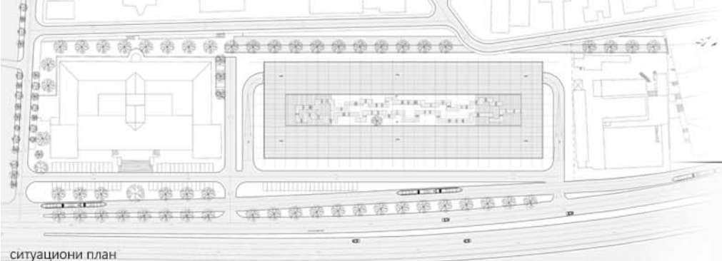
ситуациони план
