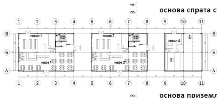
основа приземља стамбеног објекта
