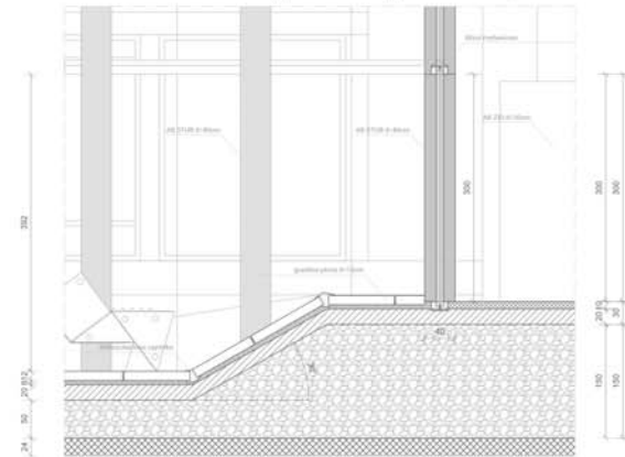
ДЕТАЉ АТРИЈУМСКОГ ДЕЛА И ДЕНИВЕЛАЦИЈЕ
