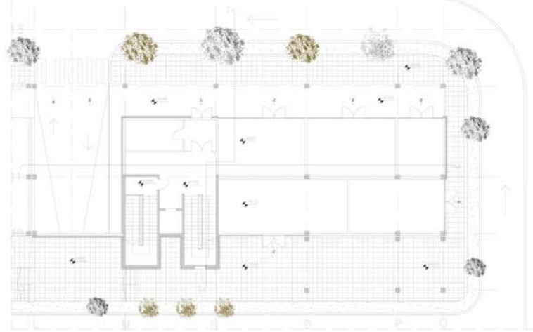
Osnova priprema za parking uređenje R 1:100
