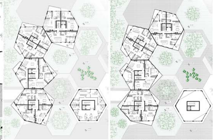
osnove stanova R 1:200
