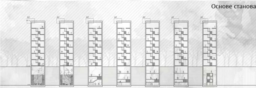
Подужни пресек
