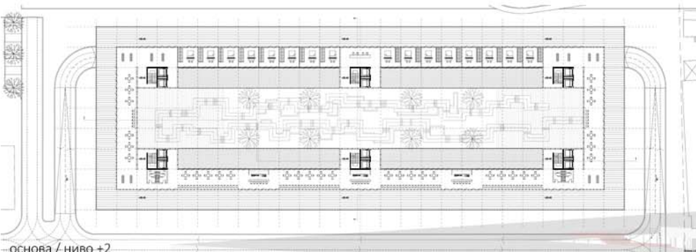
основа / ниво +2
