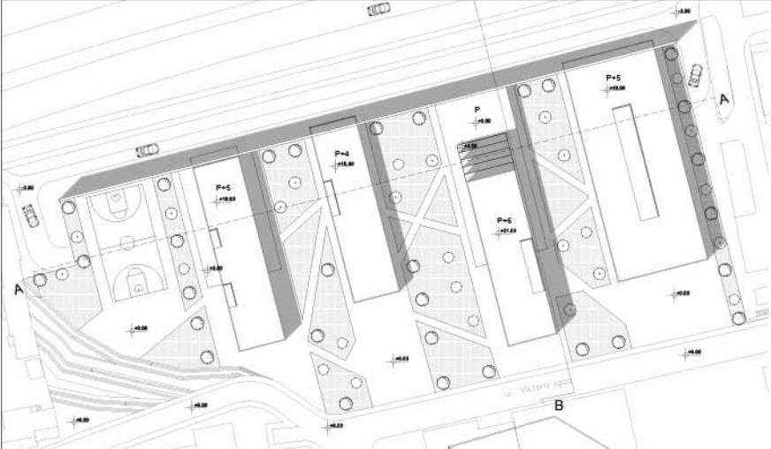
СИТУАЦИЈА
