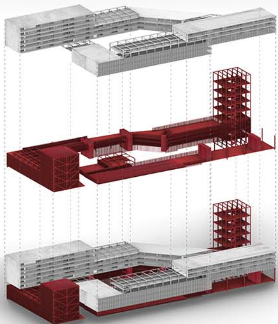
експлодирана аксонометрија
