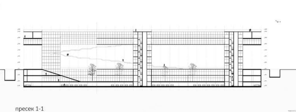
пресек 1-1
