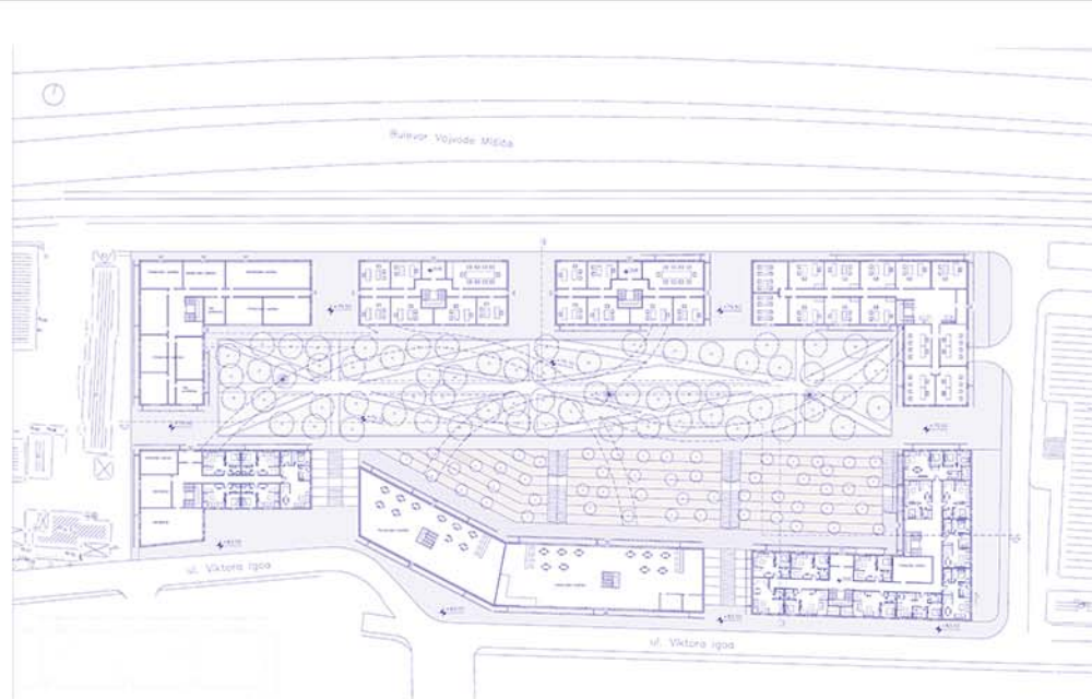
основна приземља са партерним решењем
