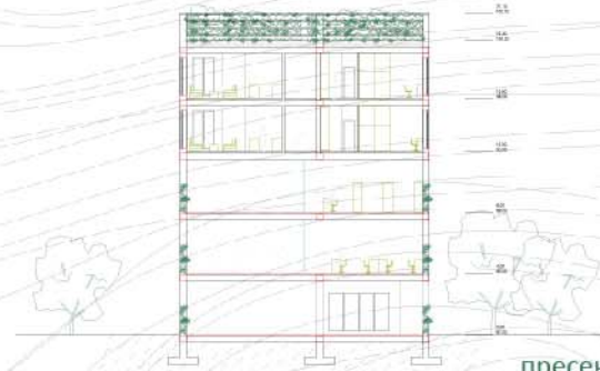
пресек 1-1
