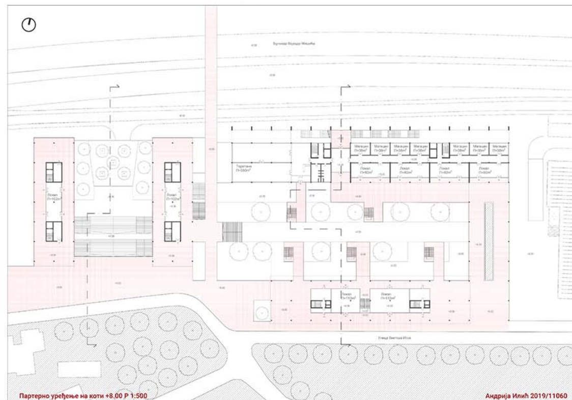
Партерно уређење на koti +8.00 P 1:500
