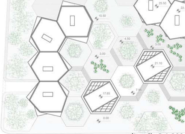
situacija R 1:200
