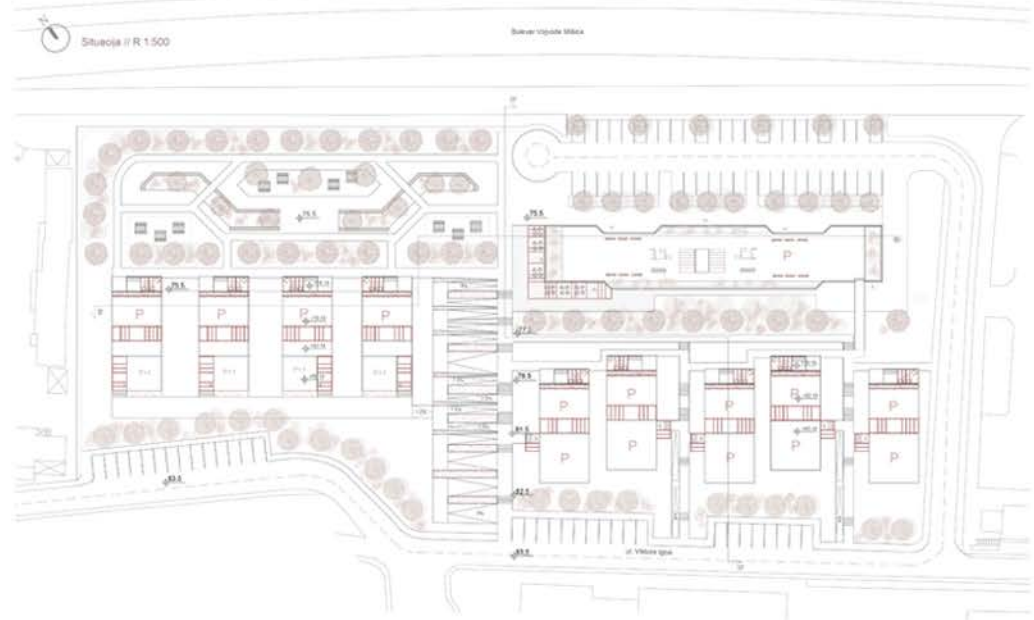
Ситуација
