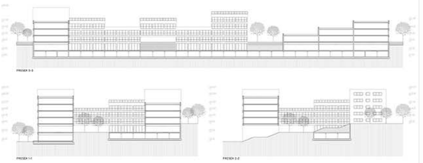
Универзитет у Београду - Архитектонски факултет/Студио 04 - Синтеза//PRESEK D1 R1:350//Prof. Doc. Milan Maksimović//Ass. Nikola Milanović//Student: SARA FILIPOVIĆ 11108_2019
