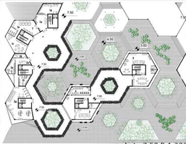
osnova kote 7.50 R 1:200
