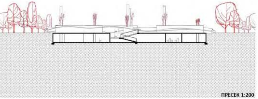
ПРЕСЕК 1:200
