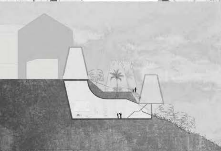
Пресек 1:50 ботаничке баште
