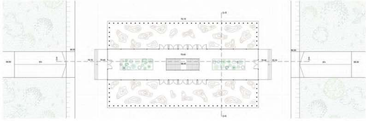
Основа приземља Р=1:100
