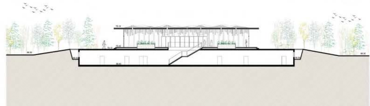
Подужни пресек Р=1:100
