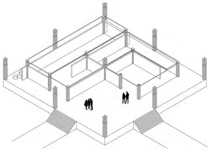
Аксонometriјски приказ Р 1:100
