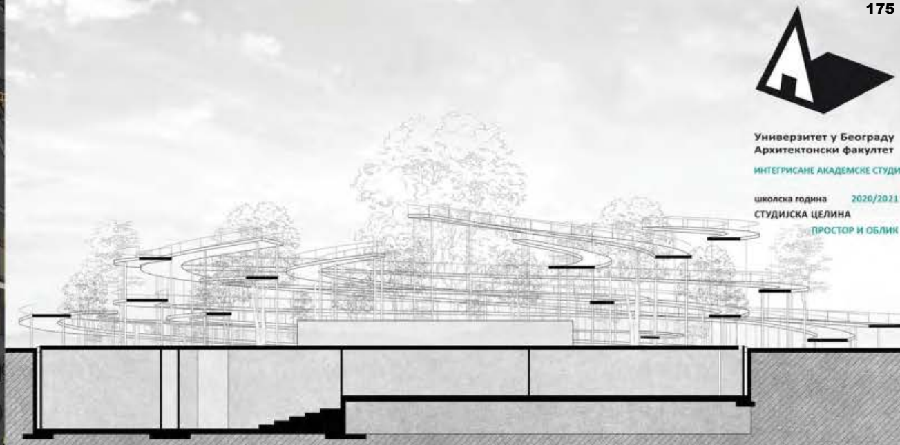
ПРЕСЕК А-А
