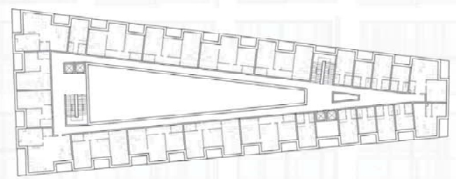
ОСНОВА ТИПСКОГ СПРАТА
