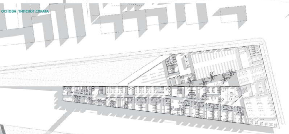
ОСНОВА ТИПСКОГ СПРАТА
