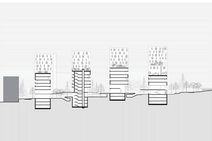
пресек 1-1
