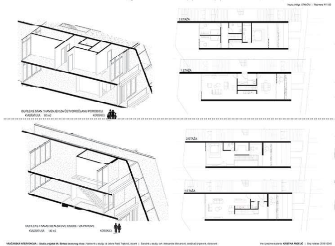
станови р1:100
