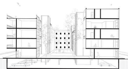
Попречни пресек кроз перспективни приказ
