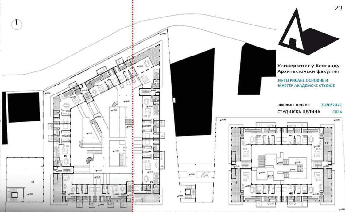
ОСНОВА ТИПСКОГ СПРАТА
