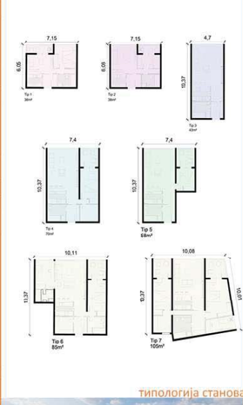
типологија станова
