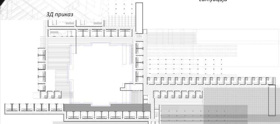
основа типског спрата P-1:300
